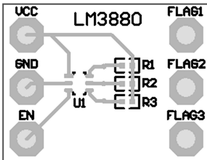
图 9-1. LM3880-Q1 顶层
