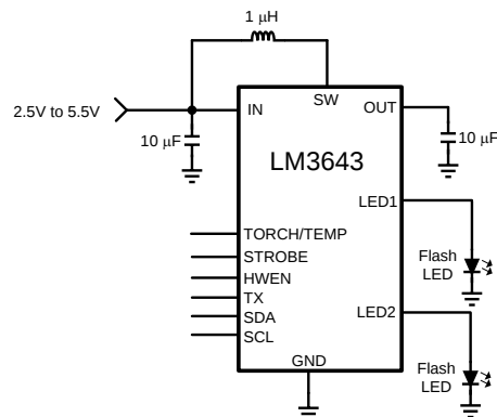
简化电路原理图
