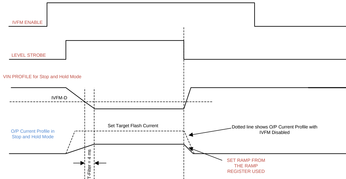
图 19. IVFM Mode
