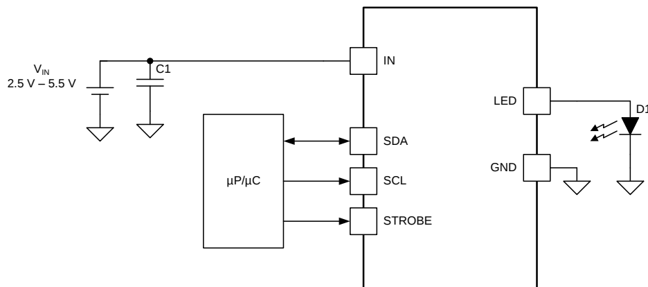
简化电路原理图
