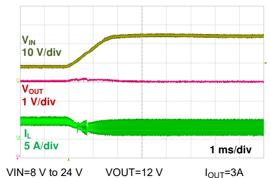
图 6-18. Line Transient
