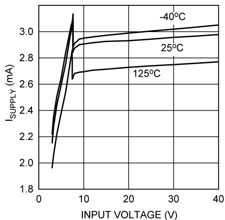
图 5-3. I_{SUPPLY} 与 V_{IN} 间的关系 (开关)
