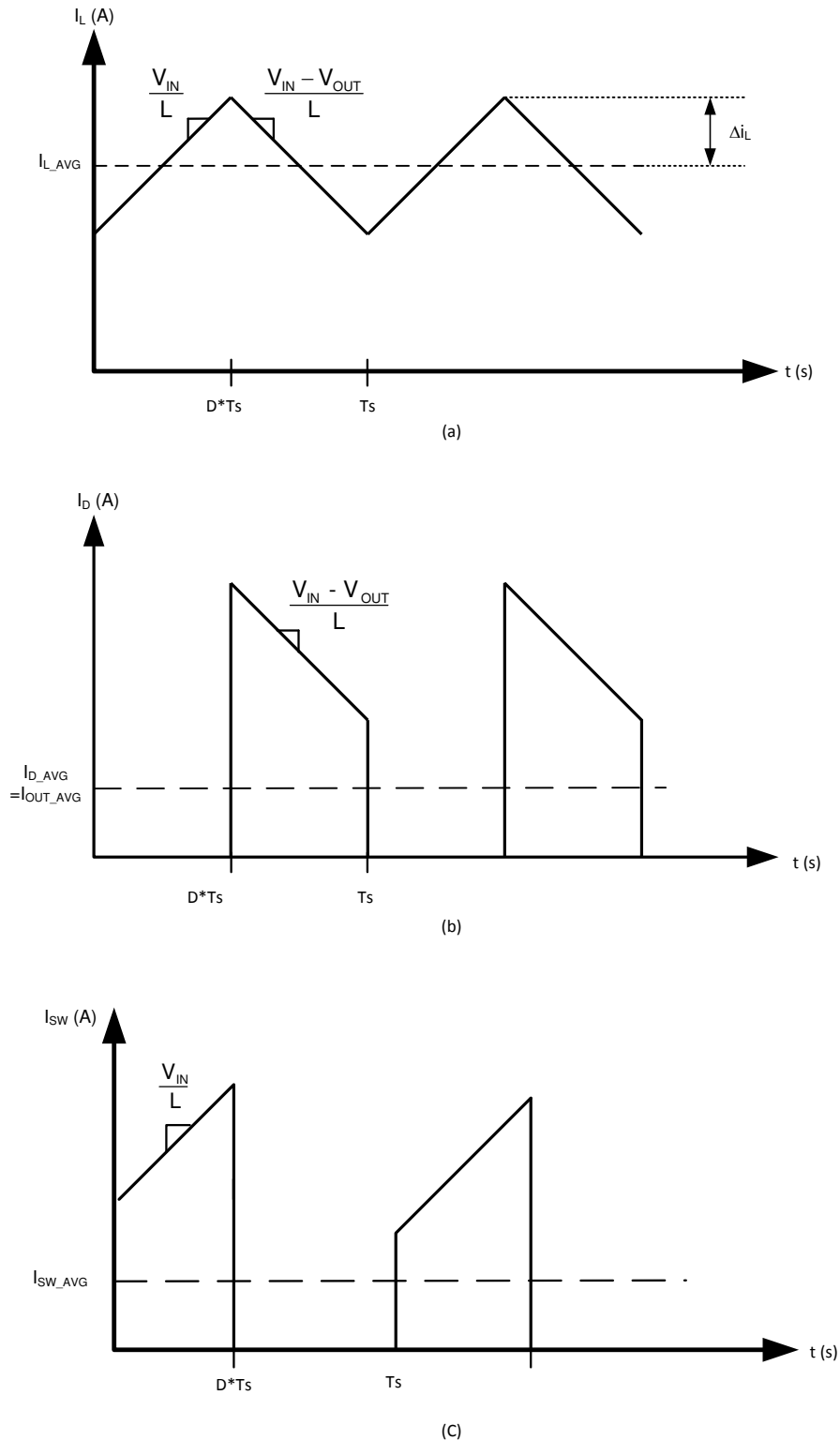
图 7-3. 电感器电流和二极管理电流
