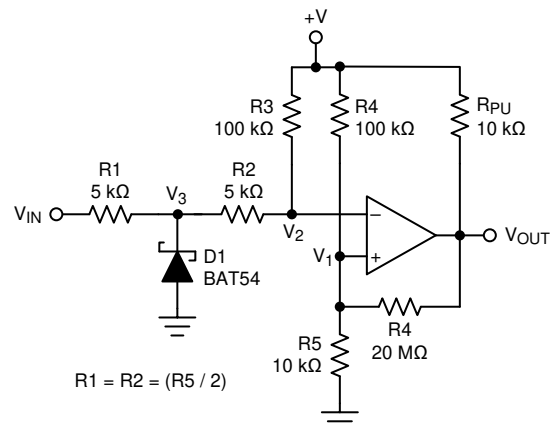
图 7-17. 过零检测器
