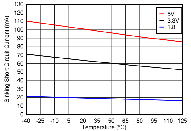
图 5-10. 短路灌电流与温度间的关系
