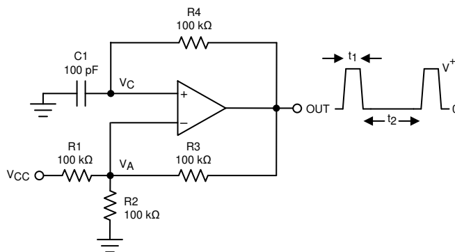
图 7-9. 方波振荡器
