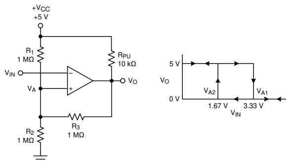
图 7-3. 具有迟滞功能的反相配置
