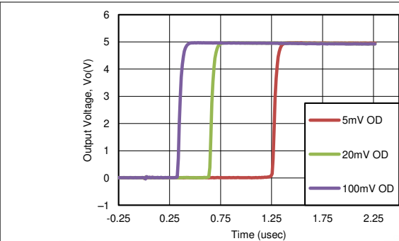
图 7-2. 各种过驱的响应时间（正转换）
