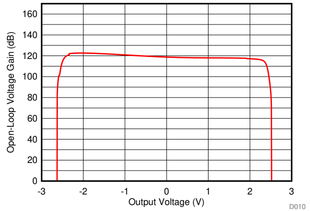
图 6-4. 开环增益与输出电压间的关系
