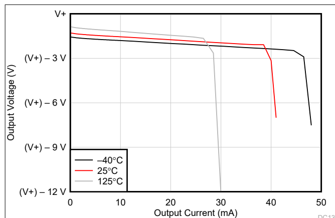
图 7-11. 输出电压摆幅与输出电流 (拉电流) 间的关系
