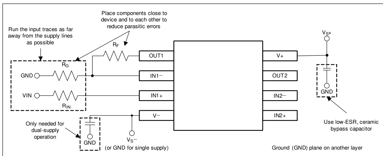
图 12-1. 同相配置的运算放大器电路板布局
