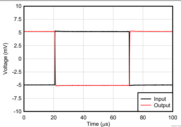
图 7-28. 过载恢复
