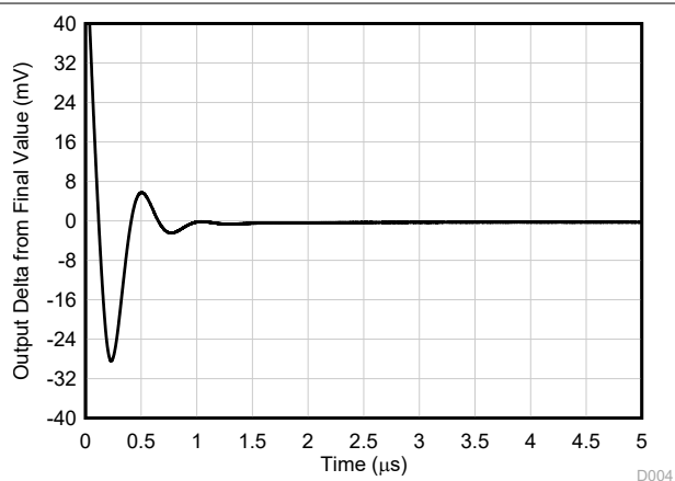
图 7-30. 小信号阶跃响应, G = -1
