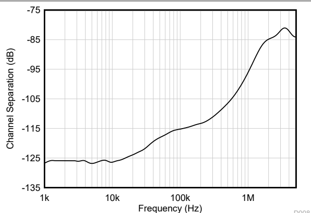
图 7-37. 通道隔离与频率间的关系
