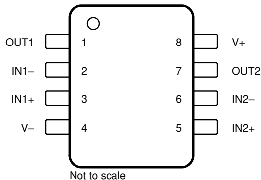
图 6-1. D、DGK 和 PW 封装 8 引脚 SOIC、VSSOP 和 TSSOP 顶视图
