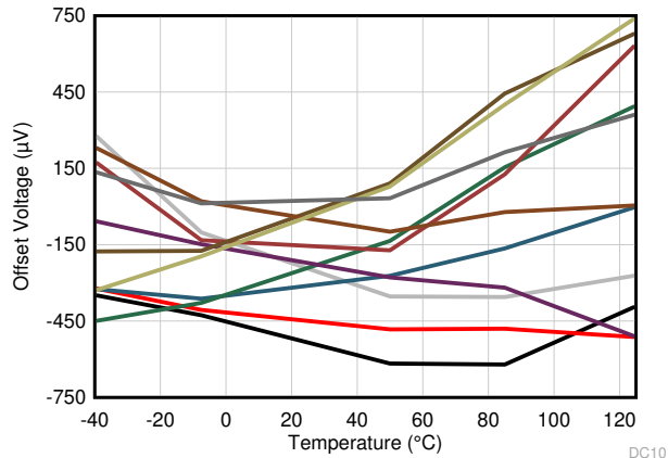
图 7-3. 失调电压与温度间的关系
