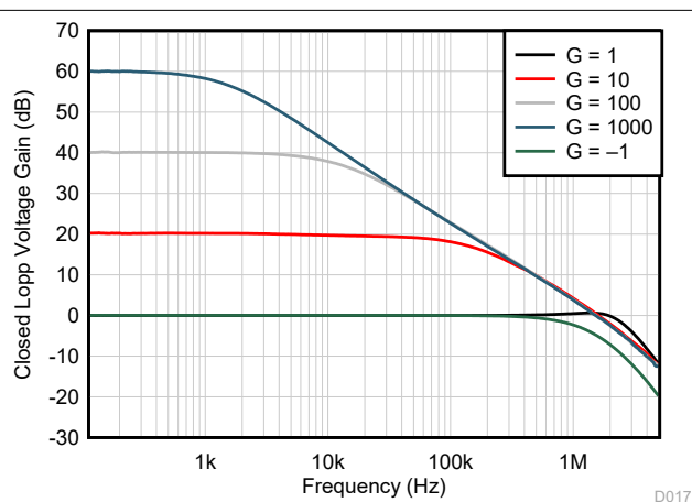
图 7-6. 闭环增益与频率间的关系
