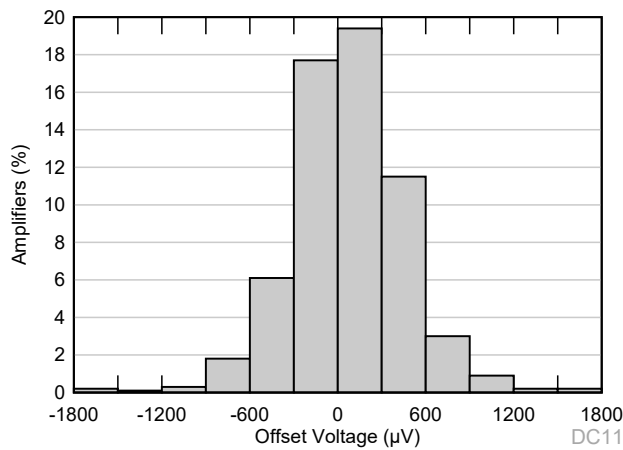
图 7-1. 失调电压生产分配
