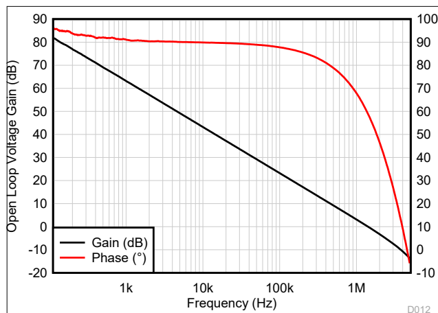
图 7-5. 开环增益和相位与频率间的关系
