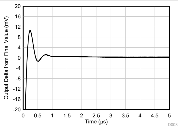
图 7-29. 小信号阶跃响应, G = 1
