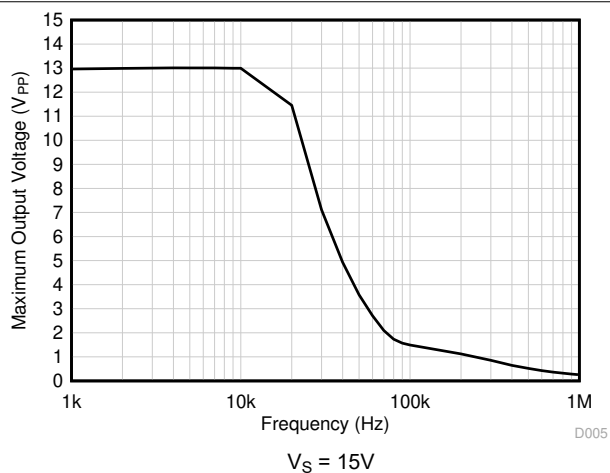
图 7-36. 最大输出电压与频率间的关系
