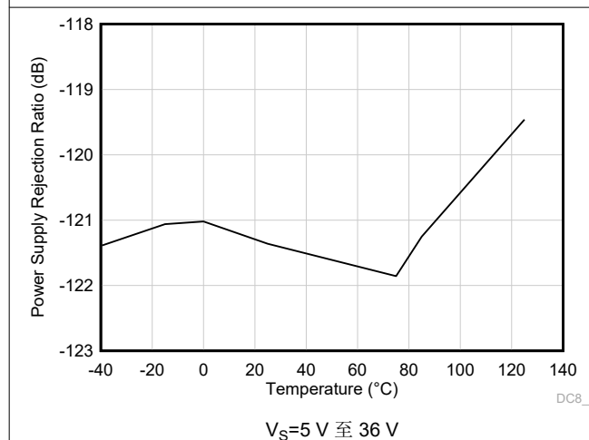
图 7-15. 电源抑制比与温度间的关系 (dB)
