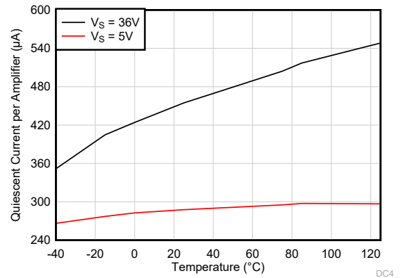
图 7-23. 静态电流与温度间的关系
