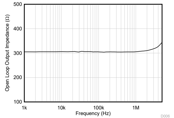
图 7-24. 开环输出阻抗与频率间的关系
