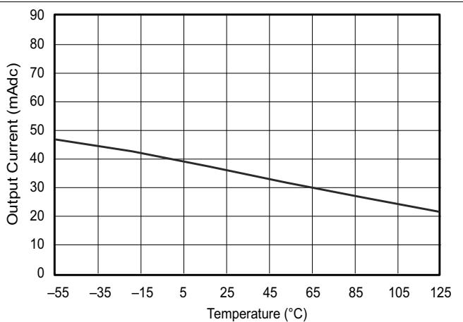
图 5-48. 拉电流限制
