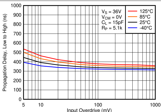
图 5-30. 低电平至高电平传播延迟与输入过驱电压之间的关系, 36V
