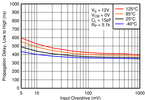
图 5-28. 低电平至高电平传播延迟与输入过驱电压之间的关系, 12V
