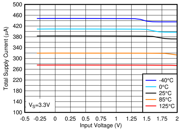
图 5-3. 3.3V 下总电源电流与输入电压之间的关系
