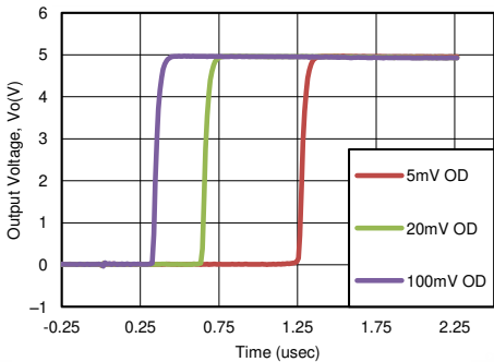
图 7-2. 各种过驱的响应时间（正转换）
