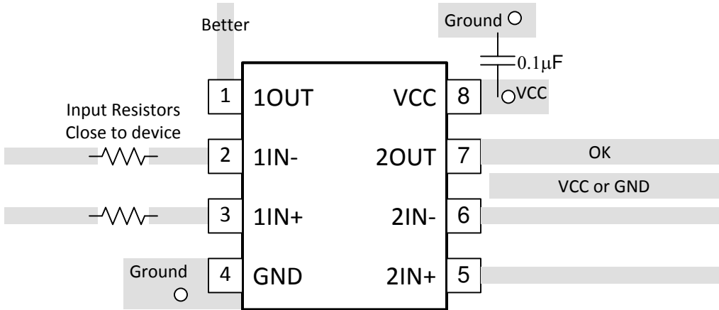
图 7-4. LM2903 布局示例
