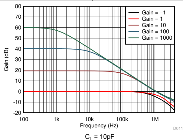
图 6-5. 闭环增益与频率间的关系
