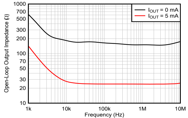
图 5-20. 开环输出阻抗与频率间的关系
