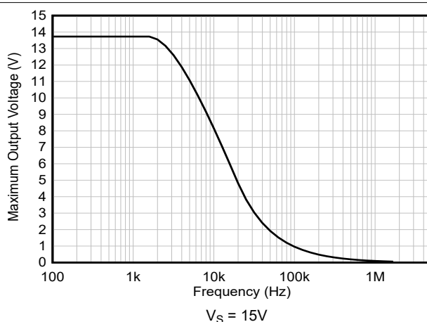
图 5-32. 最大输出电压与频率间的关系
