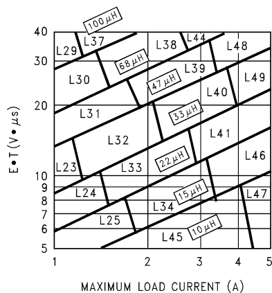
图 7-5. LM2678 可调节
