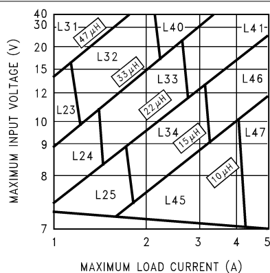
图 7-3. LM2678-5
