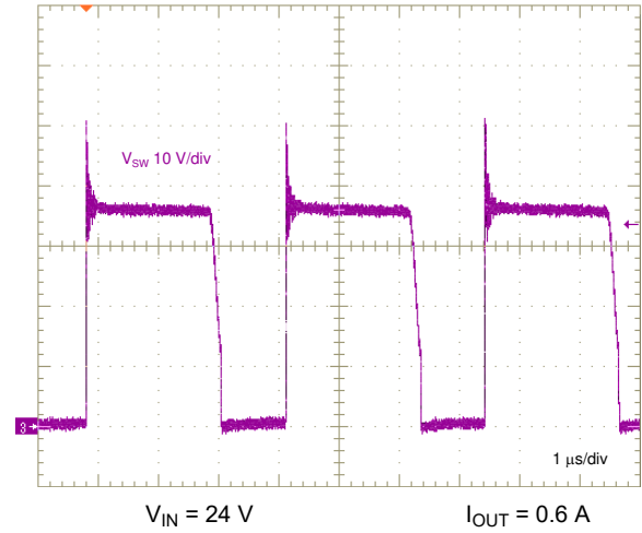
图 8-9. Switch Node Voltage
