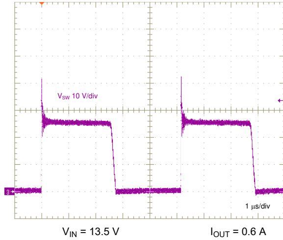
图 8-8. Switch Node Voltage
