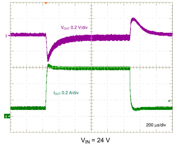
图 8-11. Load Transient, 0.1 A to 0.6 A, 0.1 A/μs
