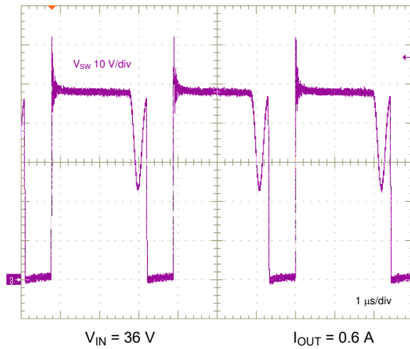
图 8-10. Switch Node Voltage
