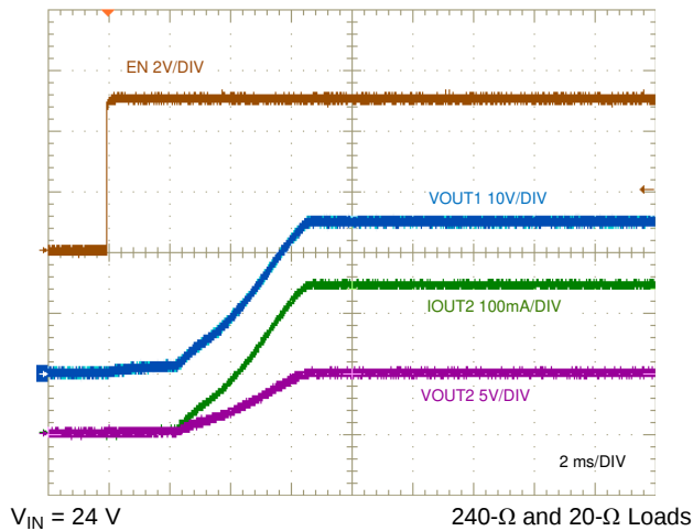
图 48. ENABLE ON Characteristic
