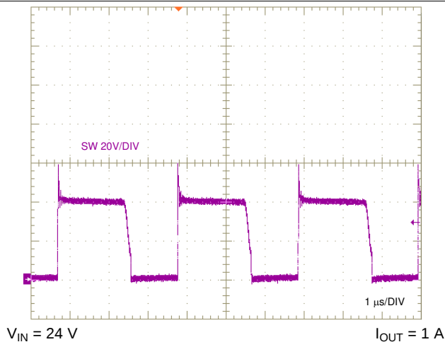
图 30. SW Node Voltage
