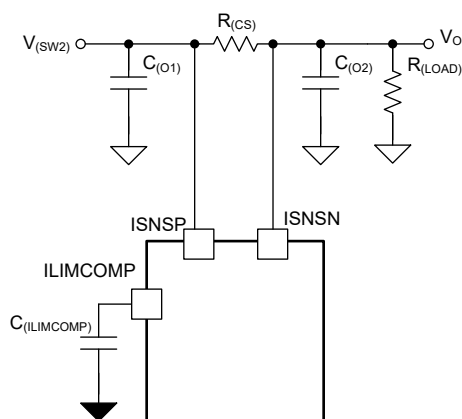
图 8-20. 具有阻性负载的电流限制元件简化版原理图
