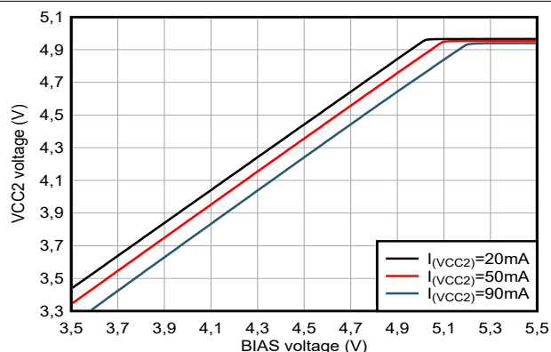
图 6-14. VCC2 LDO 输出电压与 BIAS 电压间的关系 V_{(VIN)} = 2.5V
