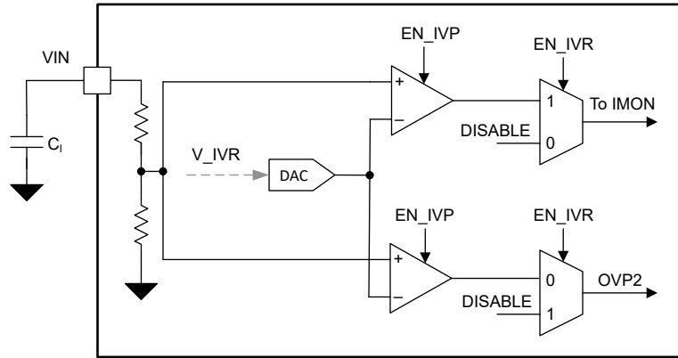
图 8-32. IVP/IVR 功能方框图
