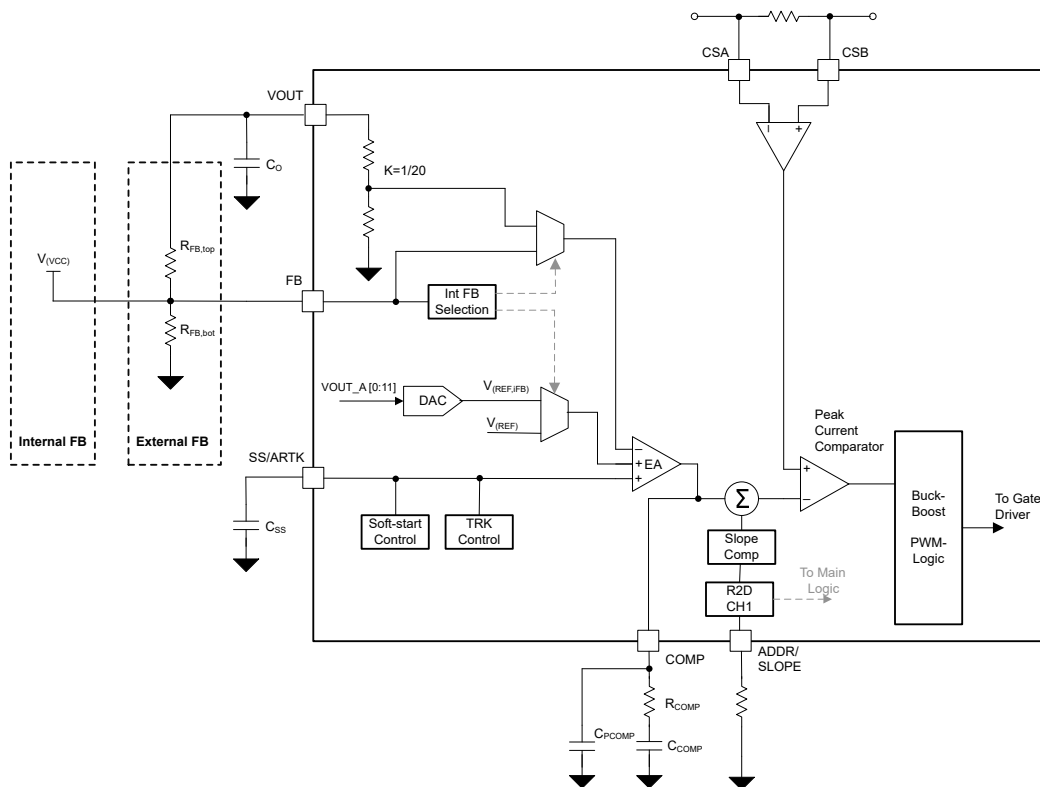
图 8-16. EA 功能方框图
