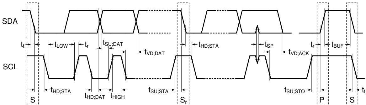
图 8-35. I 2 C 数据传输时序
