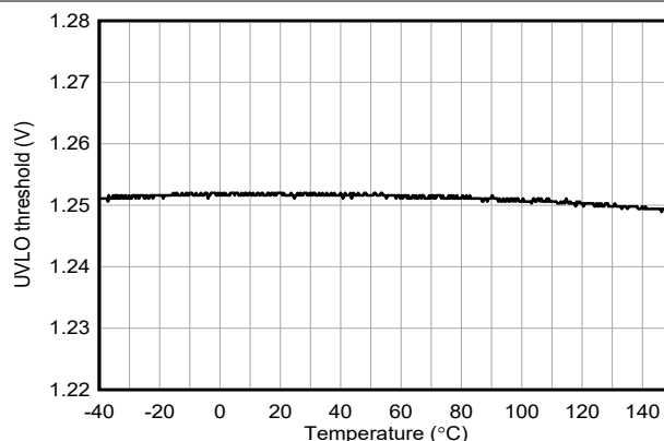
图 6-16. EN/UVLO 阈值与温度间的关系
