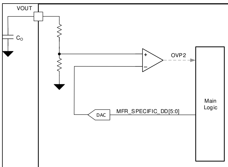
图 8-31. OVP2 功能方框图
