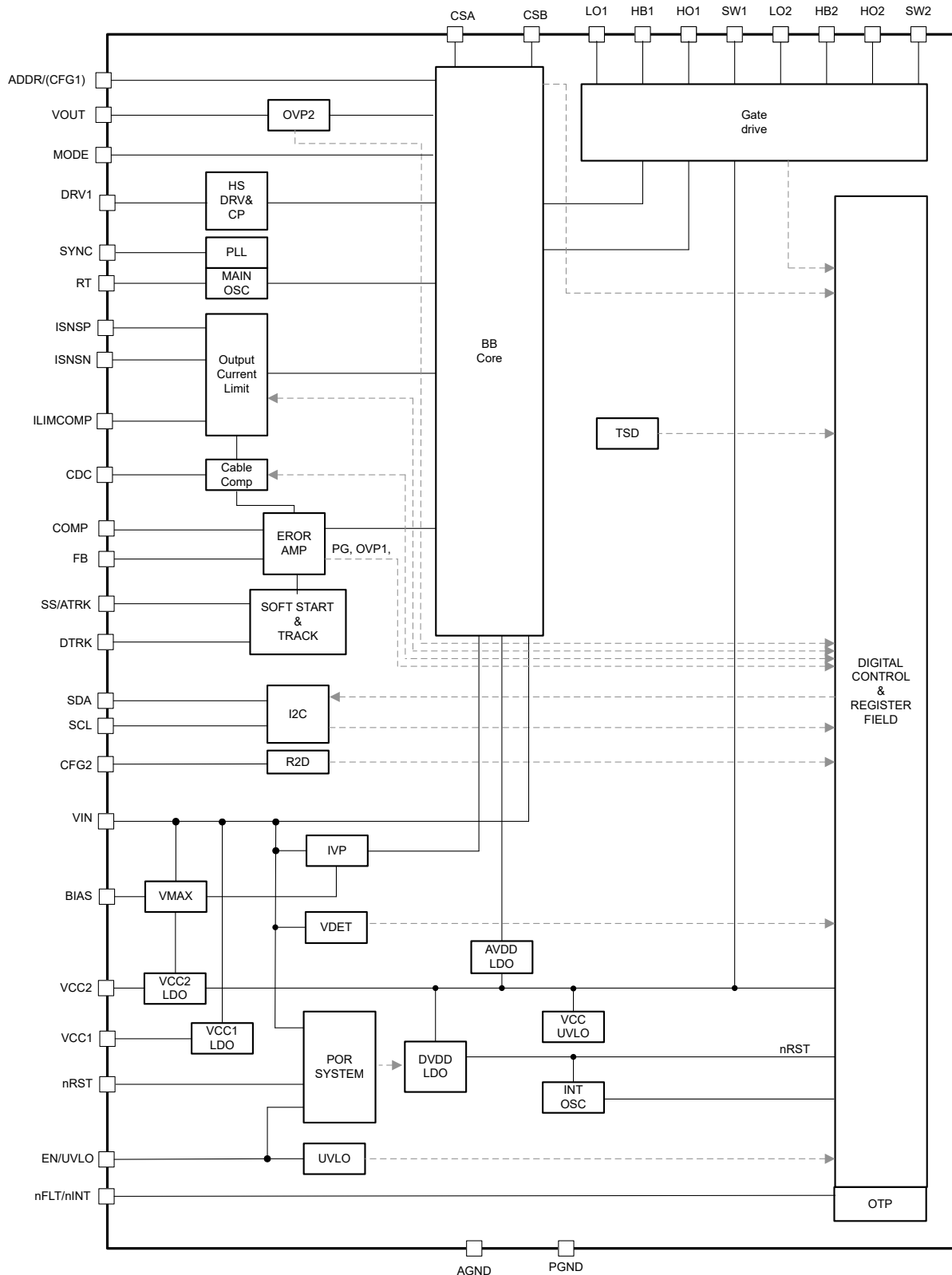
图 8-1. LM251772-Q1 功能方框图
