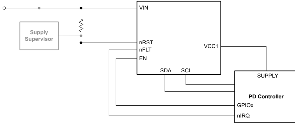
图 8-13. 简化版原理图
