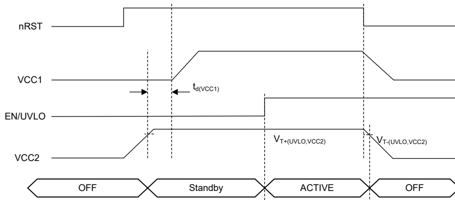
图 8-14. VCC 稳压器时序图
