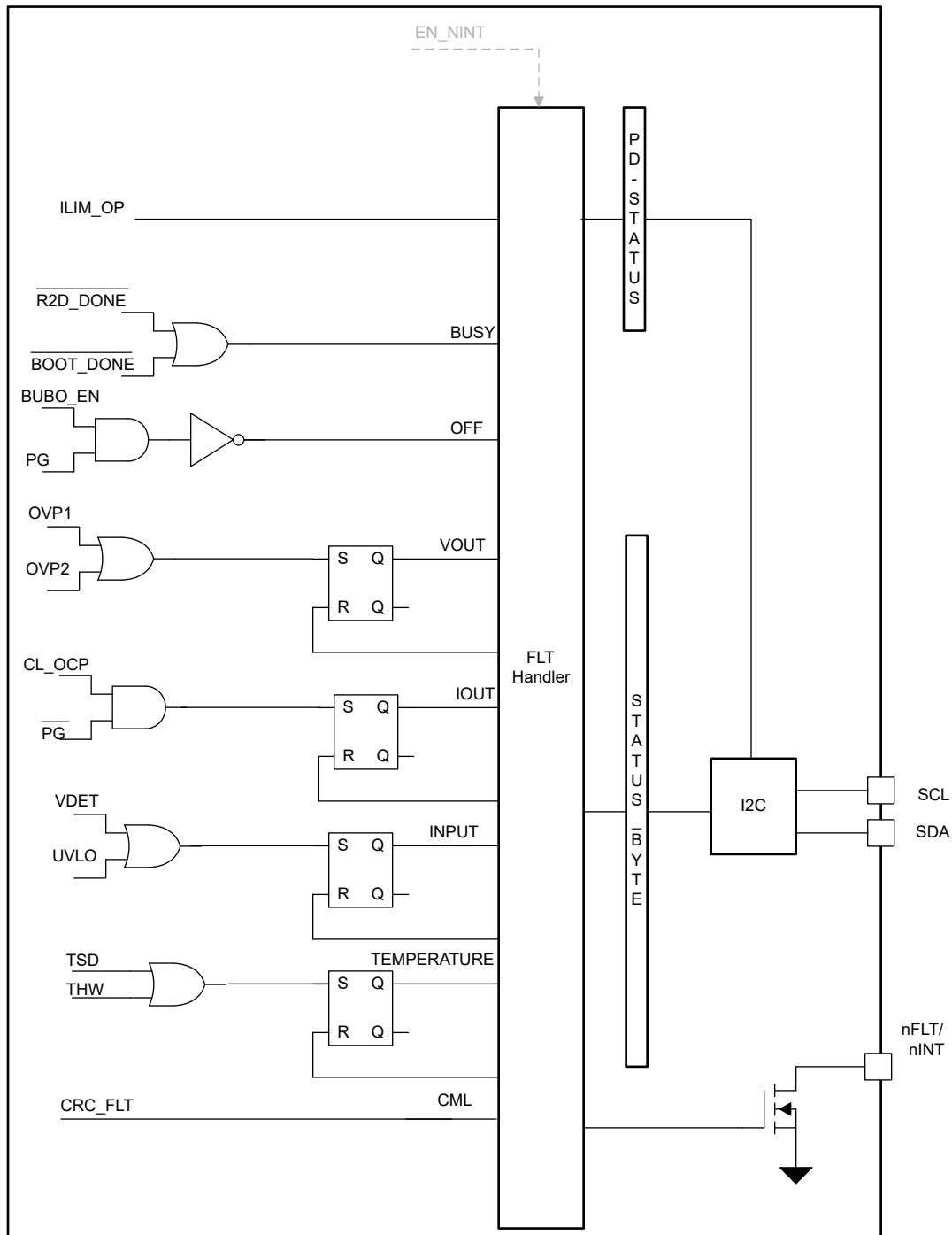
图 8-30. 功能方框图故障处理程序
