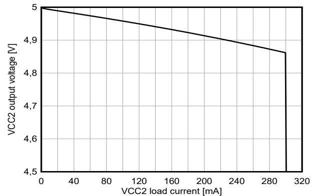
图 6-12. VCC2 LDO 输出电压与 VCC2 负载电流间的关系 V_{(VIN)} = 3.5\text{V} , V_{(BIAS)} = 12\text{V}
