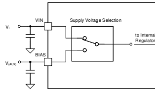
图 8-11. VSMART 电源方案 2
