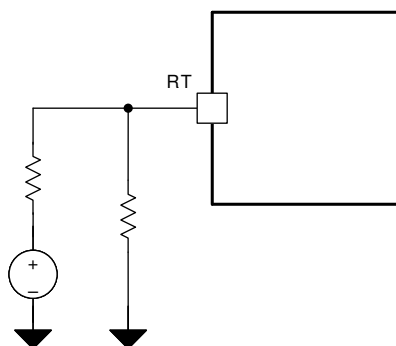
图 8-22. 动态更改频率的示例
