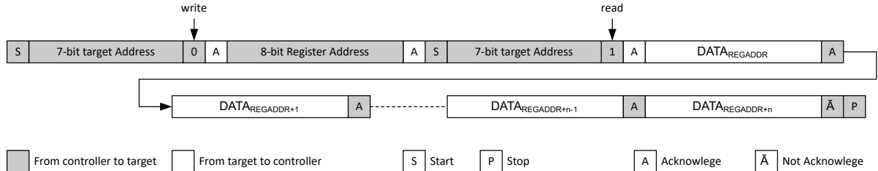
图 8-38. 从定义的寄存器地址开始进行顺序读取
