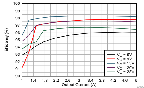
效率与输出电流间的关系， V_1 = 12V ，PSM
