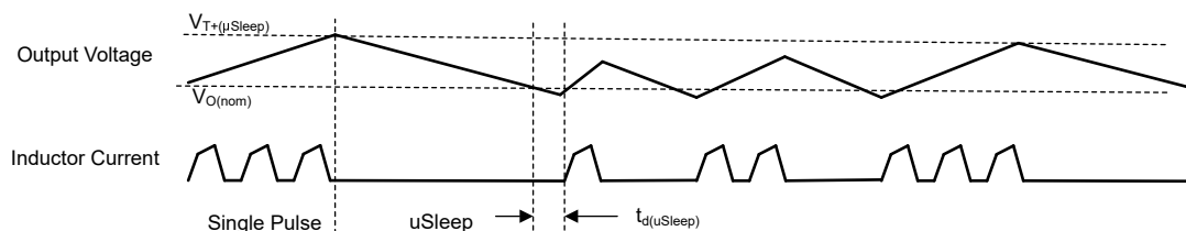
图 8-7. 省电模式的时序图 ( \mu\text{Sleep} 启用 )
