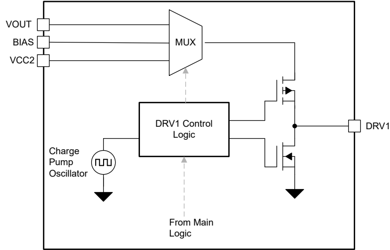
图 8-26. 功能方框图 - DRV 引脚
