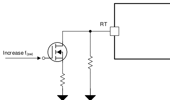
图 8-21. 跳频示例
