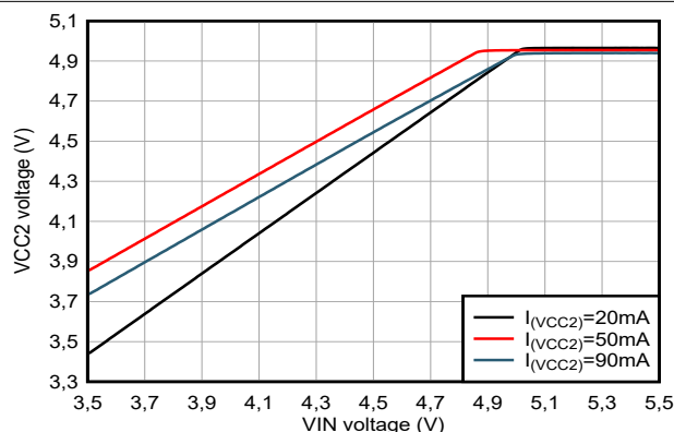
图 6-13. VCC2 LDO 输出电压与 VIN 电压间的关系 V_{(BIAS)} = 0V
