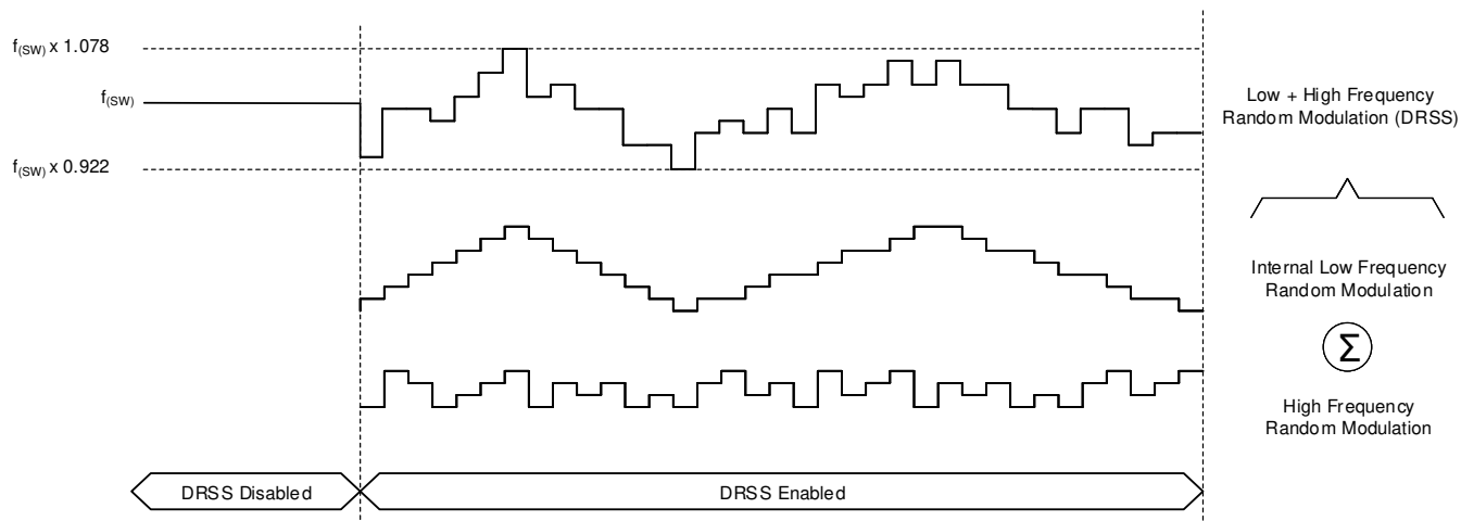
图 8-27. 双随机展频
