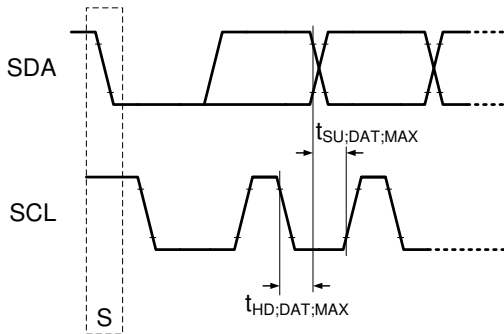
图 8-36. 最长上升/下降时间的 I 2 C 数据传输时序
