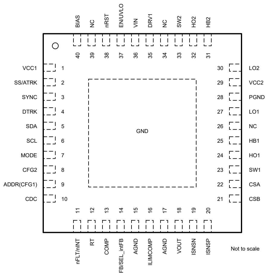
图 5-1. LM251772-Q1 RHA 封装，40 引脚 QFN (顶视图)
