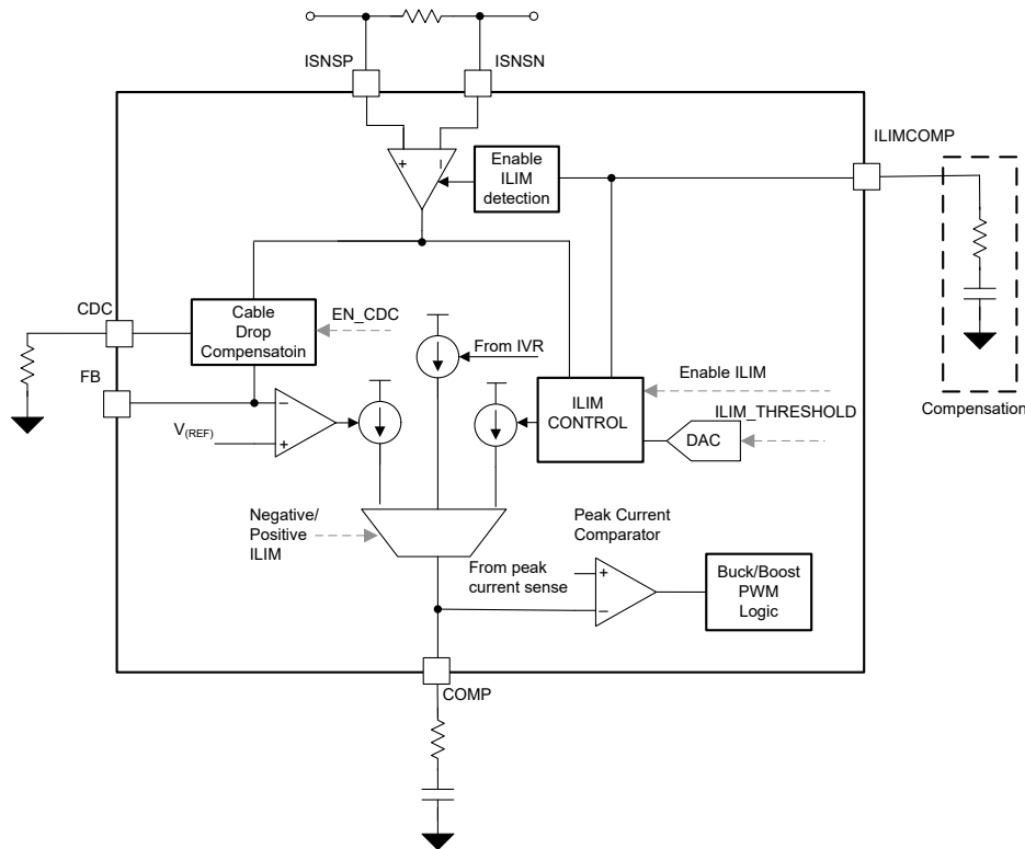
图 8-19. 电流监测功能方框图
