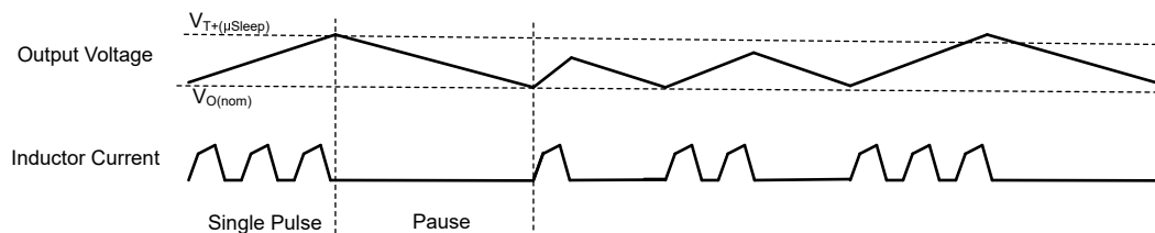
图 8-6. 省电模式的时序图 ( \mu\text{Sleep} 禁用 )
