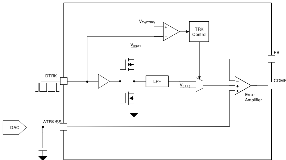
图 8-25. 输出电压跟踪功能方框图
