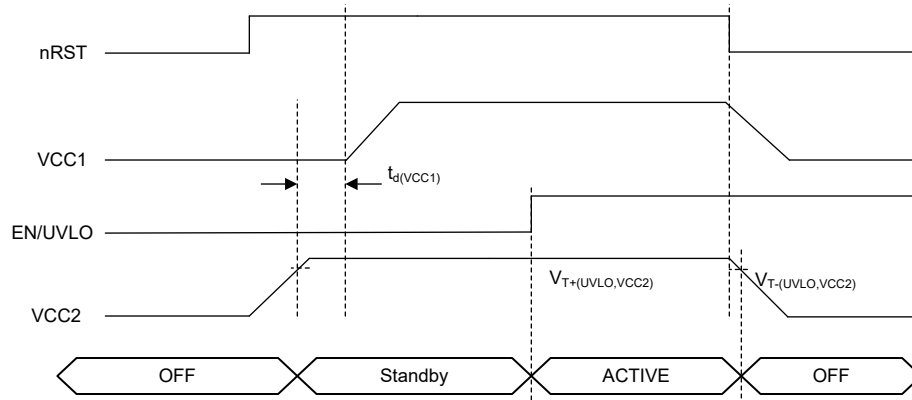
图 8-15. VCC 稳压器时序图
