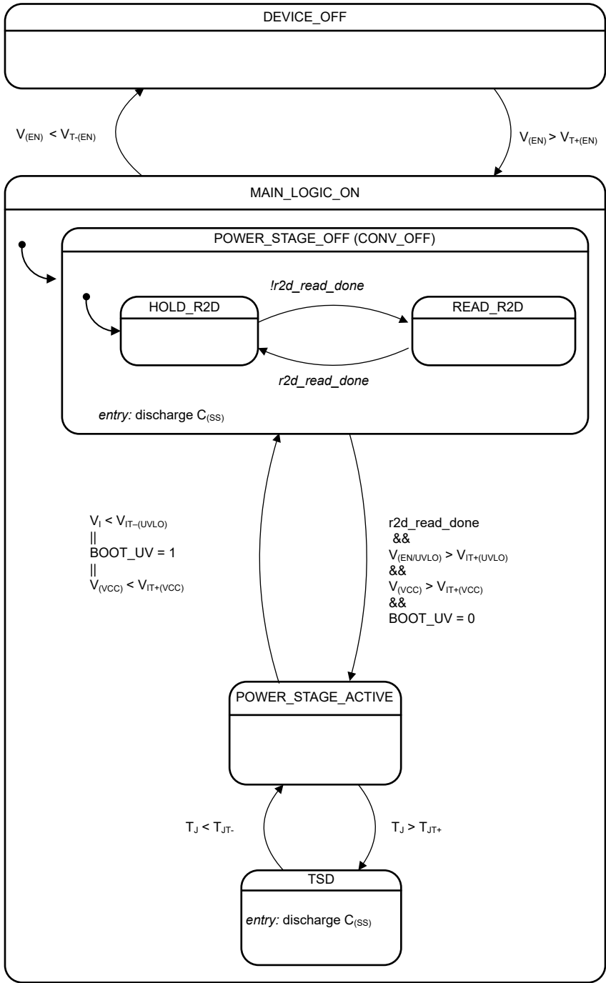
图 8-34. 状态图
