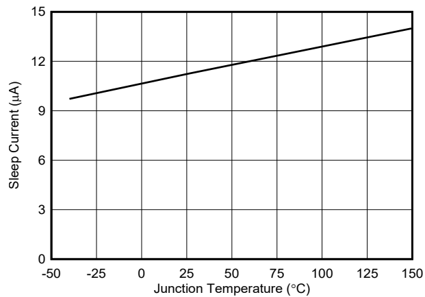
图 7-6. Sleep Current vs Temperature
