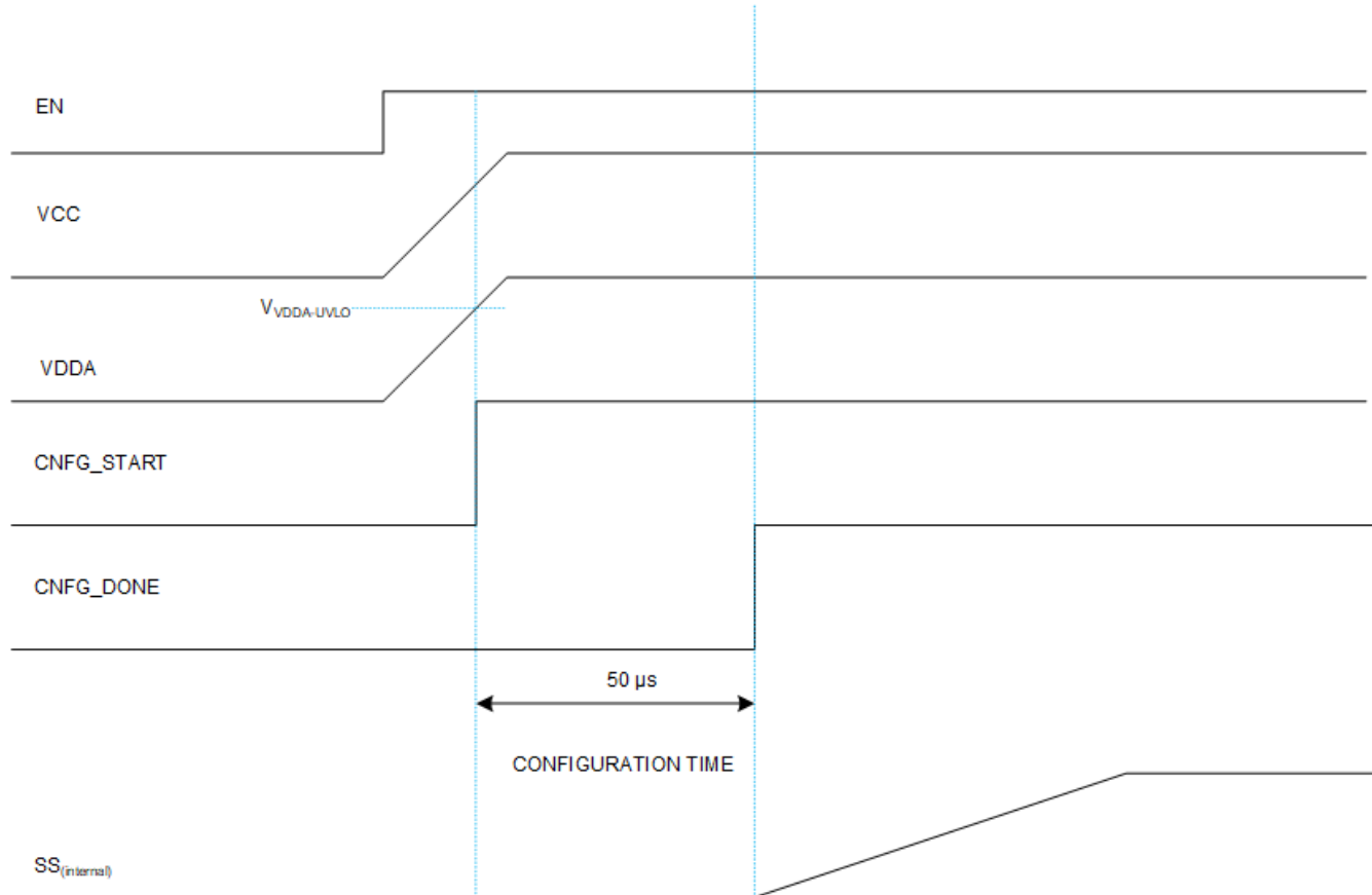
图 8-6. Configuration Timing
