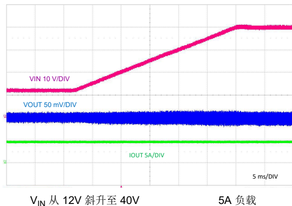
图 9-22. V_{IN} = 40V 时的线路瞬态响应
