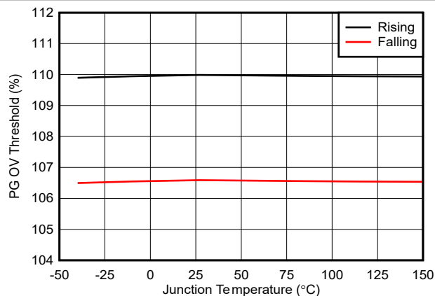
图 7-9. PG OV 阈值与温度间的关系
