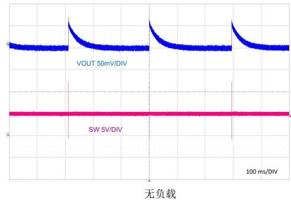
图 9-21. PFM 开关
