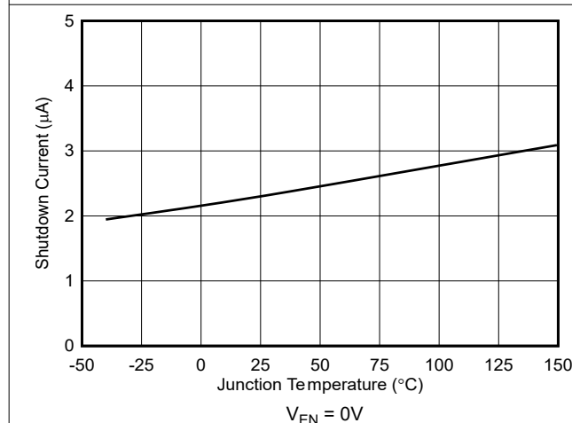
图 7-3. 关断电流与温度间的关系
