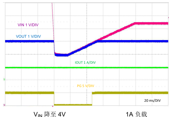
图 9-23. V_{IN} = 4V 时的线路瞬态响应
