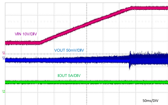
图 9-7. 满负载开关
