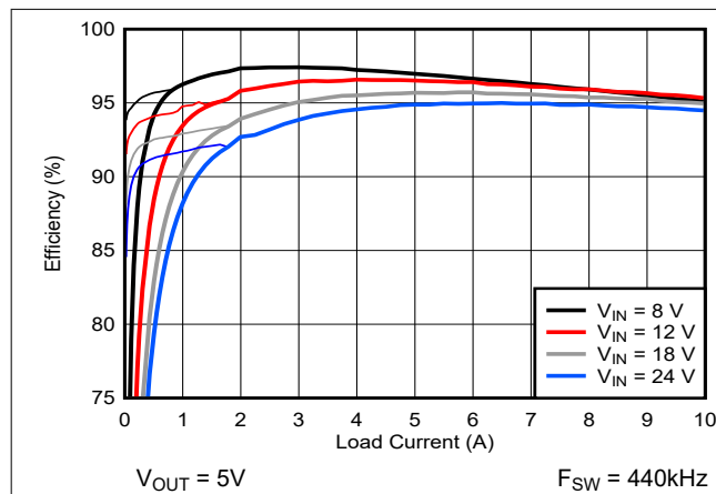
图 7-1. 效率与负载间的关系
