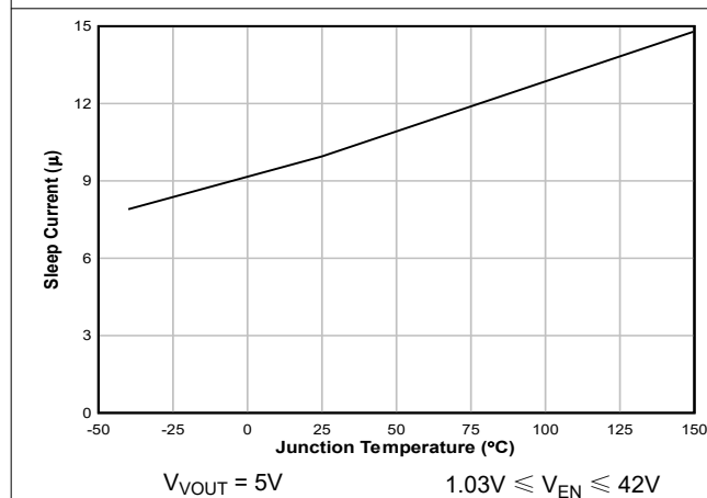
图 7-5. Sleep2 电流与温度间的关系
