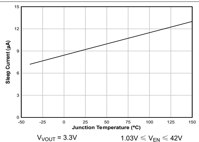
图 7-4. Sleep1 电流与温度间的关系
