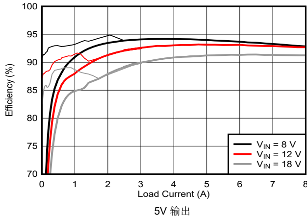
图 9-5. 效率与 I_{OUT} 之间的关系
