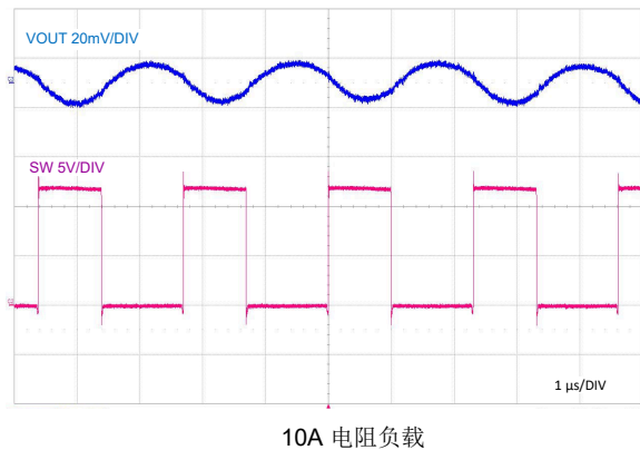
图 9-20. 满负载开关
