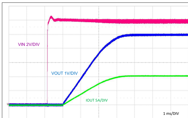
图 9-24. 启动特性
