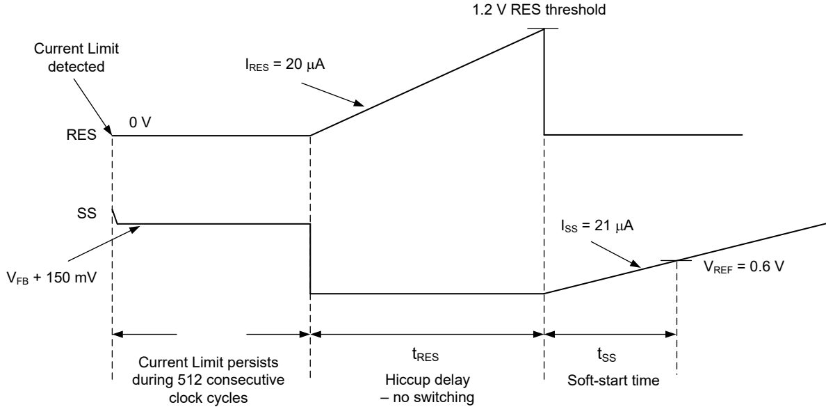
图 9-6. 断续模式时序图
