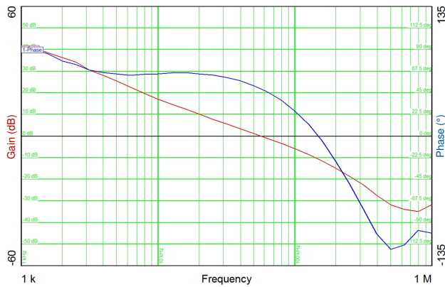
图 10-17. 波特图, 3.3V 输出
