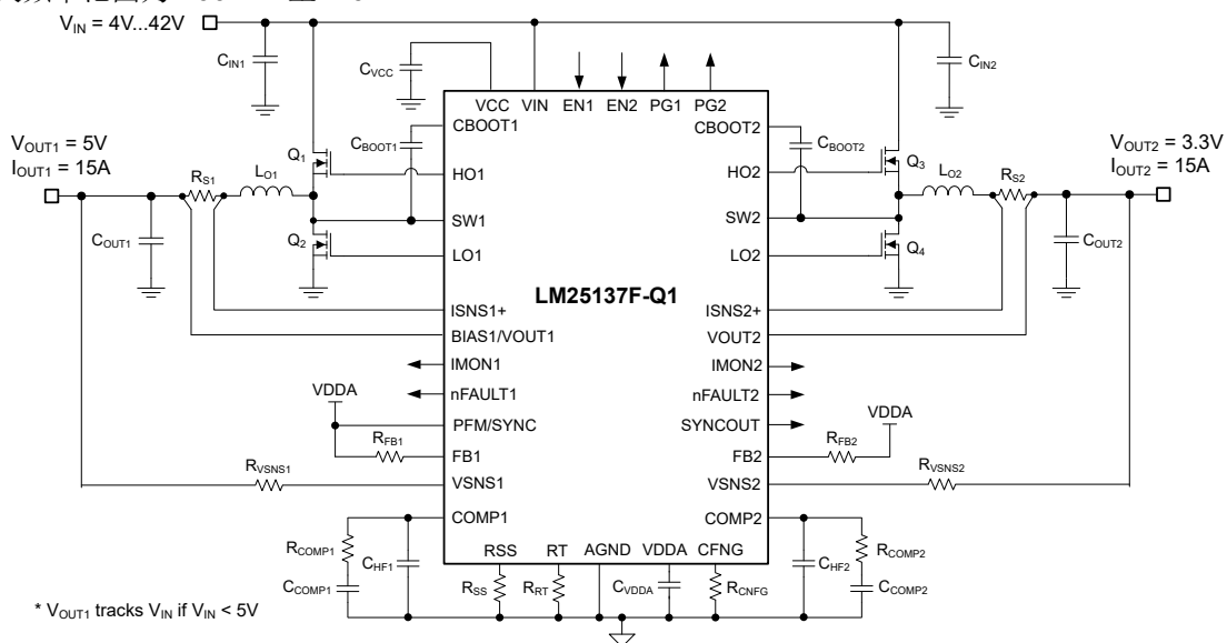
LM25137F-Q1 双路输出降压开关稳压器 - 简化原理图
