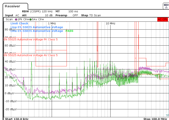
图 8-17. CISPR 25 5 类 EMI 性能，两个输出的负载为 15A
