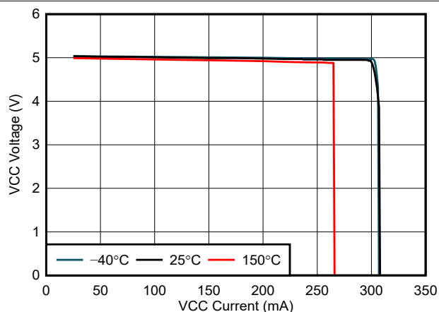
图 6-18. VCC 电流限值与温度间的关系
