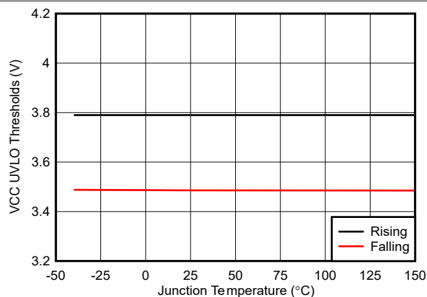
图 6-17. VCC UVLO 阈值与温度间的关系
