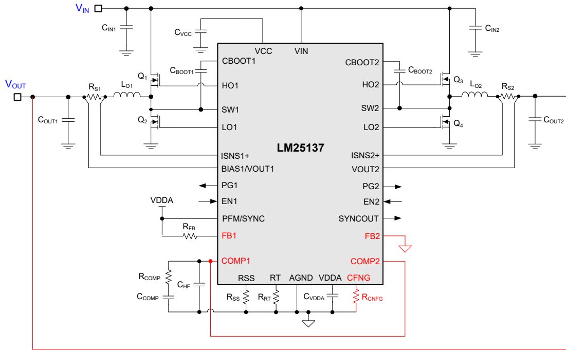
图 7-8. LM25137 配置为单输出交错式操作时的两相稳压器原理图
