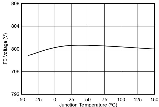
图 6-14. 反馈电压与温度之间的关系
