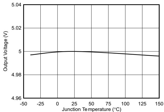
图 6-12. 固定 5V 输出电压与温度间的关系
