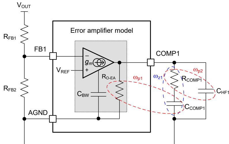
图 8-3. 电压环路误差放大器和补偿网络
