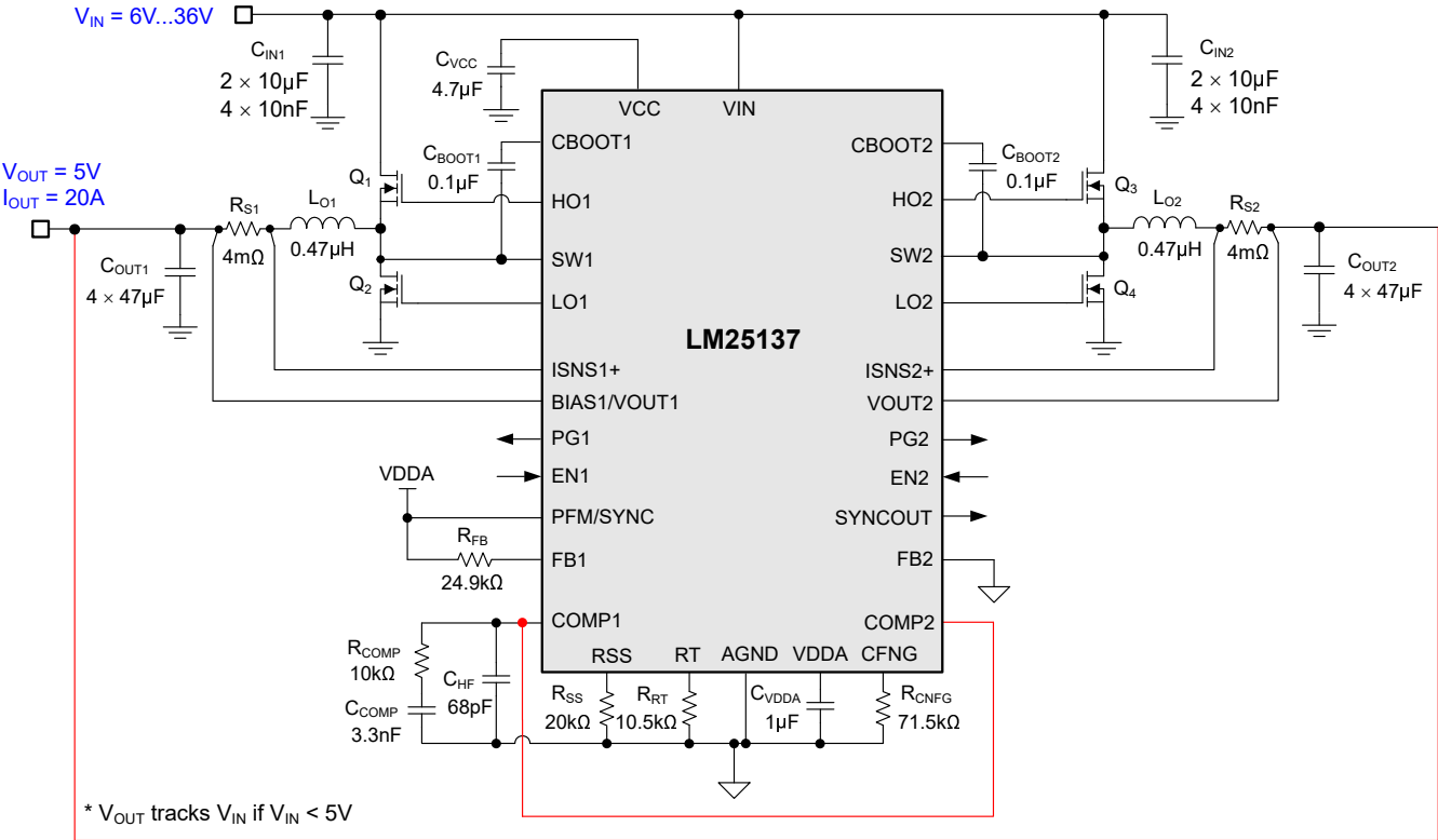
图 8-19. 采用 LM25137 两相降压稳压器且开关频率为 2.1MHz 时的应用电路 2
