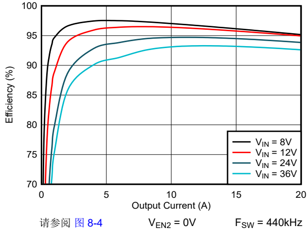
图 6-1. 效率与负载间的关系，5V 输出
