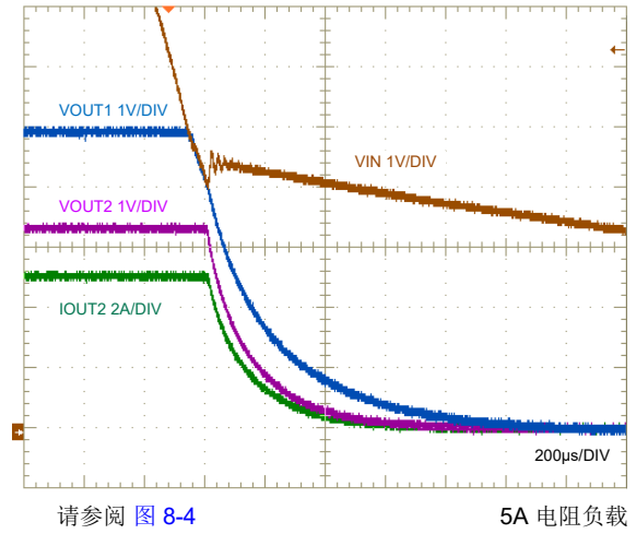
图 6-4. 关断特性
