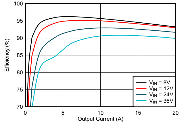
图 8-6. 效率与 I_{OUT2} 之间的关系
