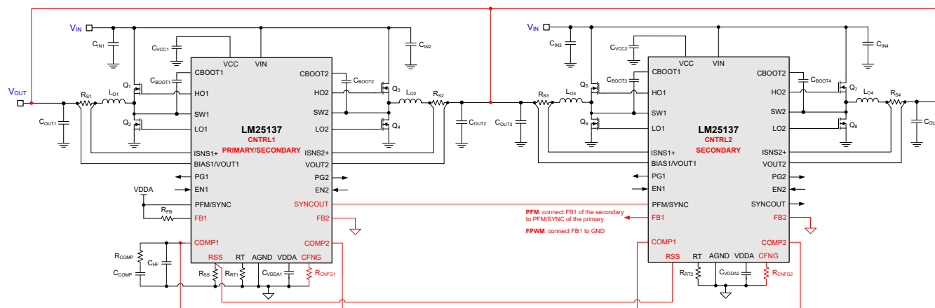
图 7-9. LM25137 配置为单输出交错式操作时的多相稳压器原理图
