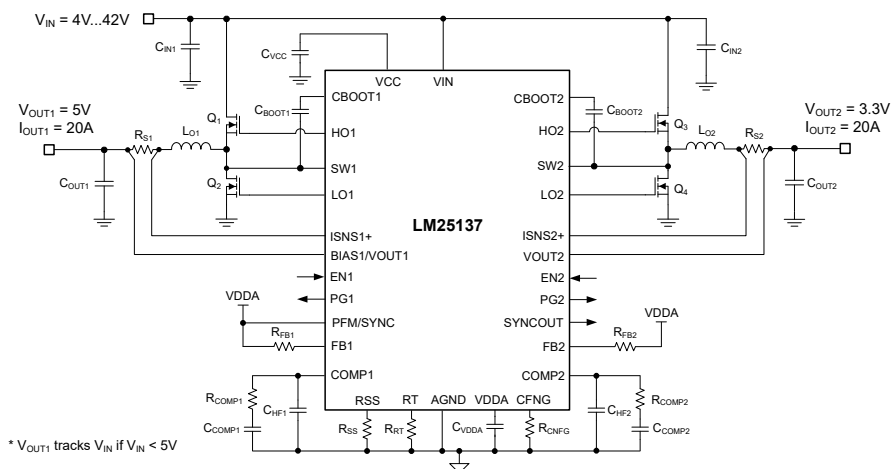
LM25137 双路输出降压开关稳压器 - 简化原理图
