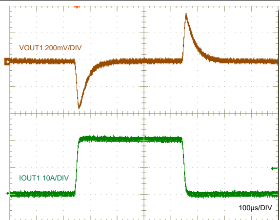
图 6-5. 负载瞬态响应
