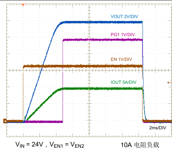
图 8-22. 使能端开启和关闭特性
