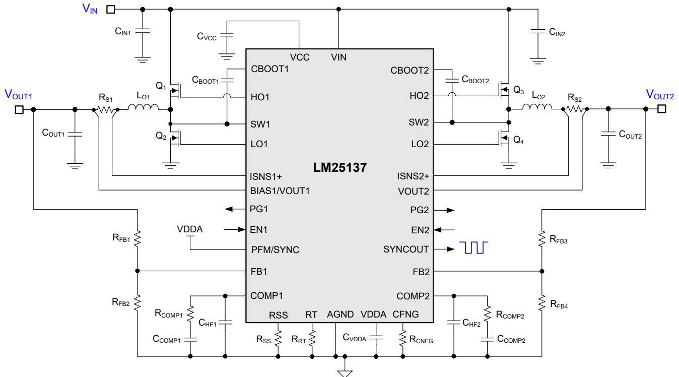
图 7-1. LM25137 双路输出稳压器原理图
