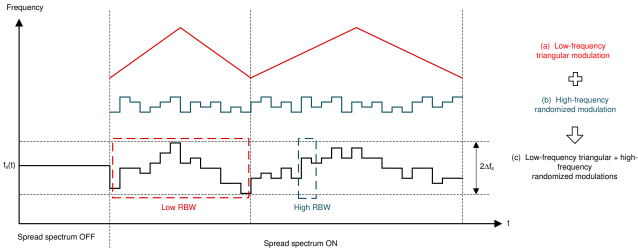
图 7-3. DRSS 实现
