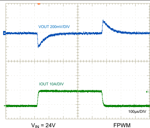
图 8-24. 负载瞬态, 0A 至 10A
