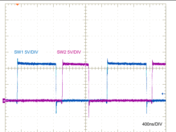
图 6-6. 开关节点电压
