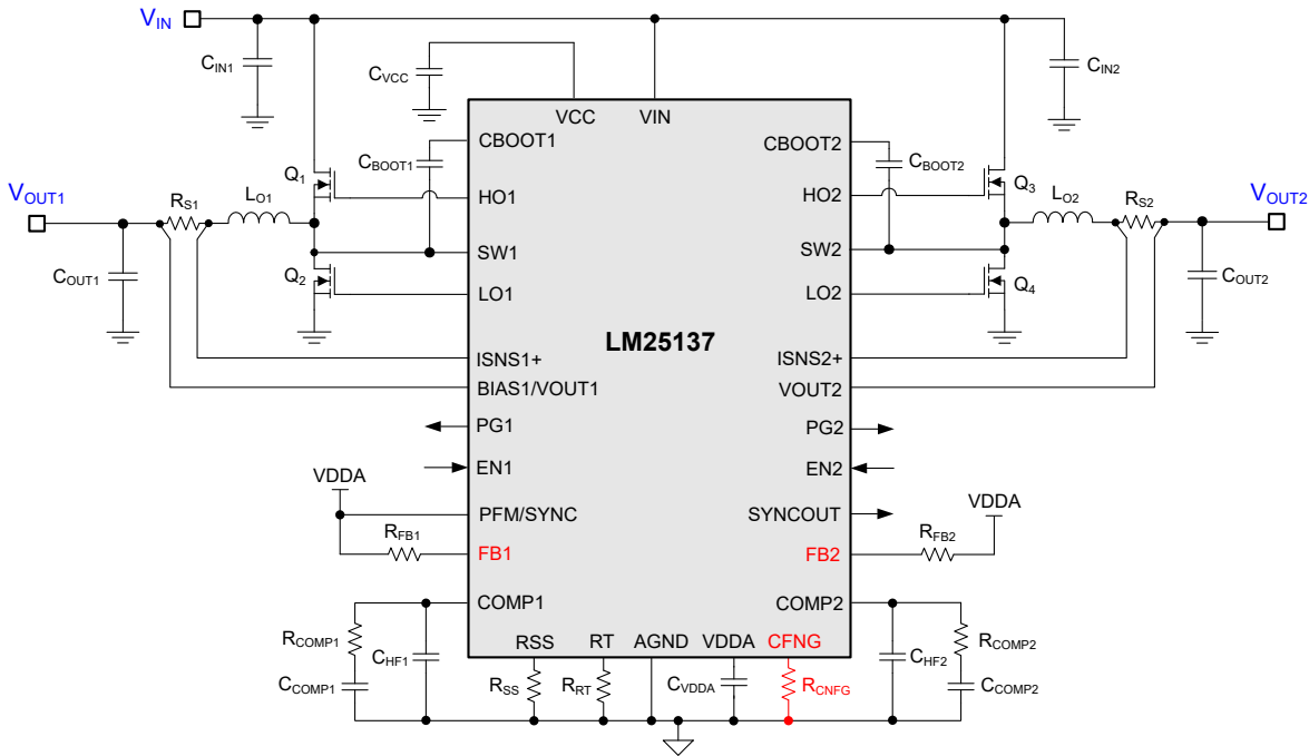
图 7-7. 为独立双路输出配置的 LM25137 稳压器原理图
