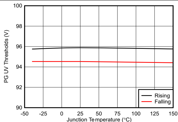
图 6-19. PG UV 阈值与温度间的关系
