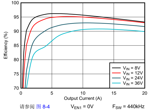
图 6-2. 效率与负载间的关系，3.3V 输出
