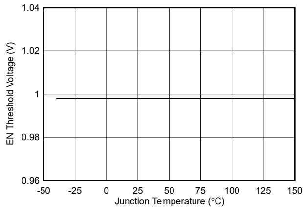
图 6-23. EN 上升阈值电压与温度间的关系
