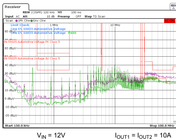
图 8-15. CISPR 25 5 类 EMI 性能，两个输出的负载为 10A
