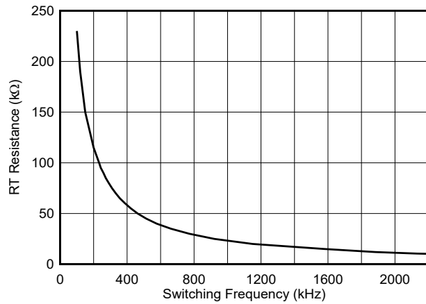
图 6-25. RT 电阻与开关频率间的关系
