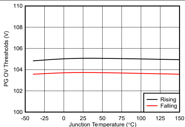
图 6-20. PG OV 阈值与温度间的关系
