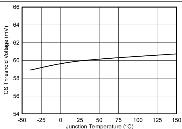
图 6-22. 电流检测阈值与温度间的关系
