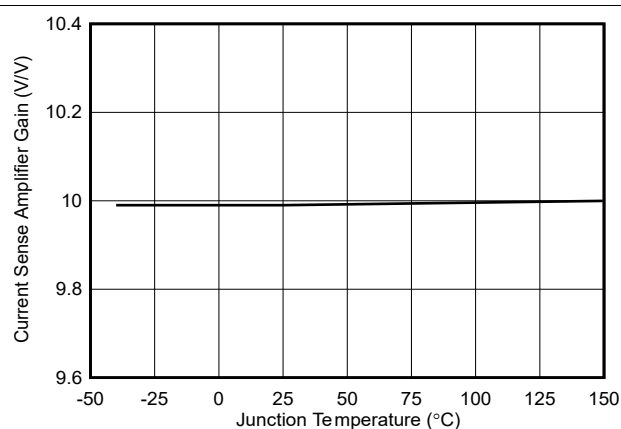
图 6-21. 电流检测放大器增益与温度间的关系
