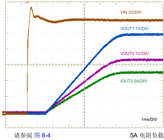
图 6-3. 启动特性
