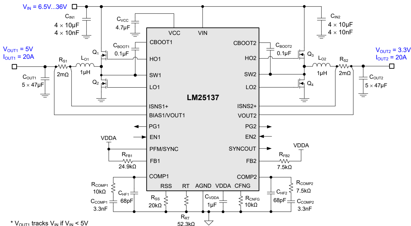
图 8-4. 采用 LM25137 降压稳压器且开关频率为 440kHz 时的应用电路 1
