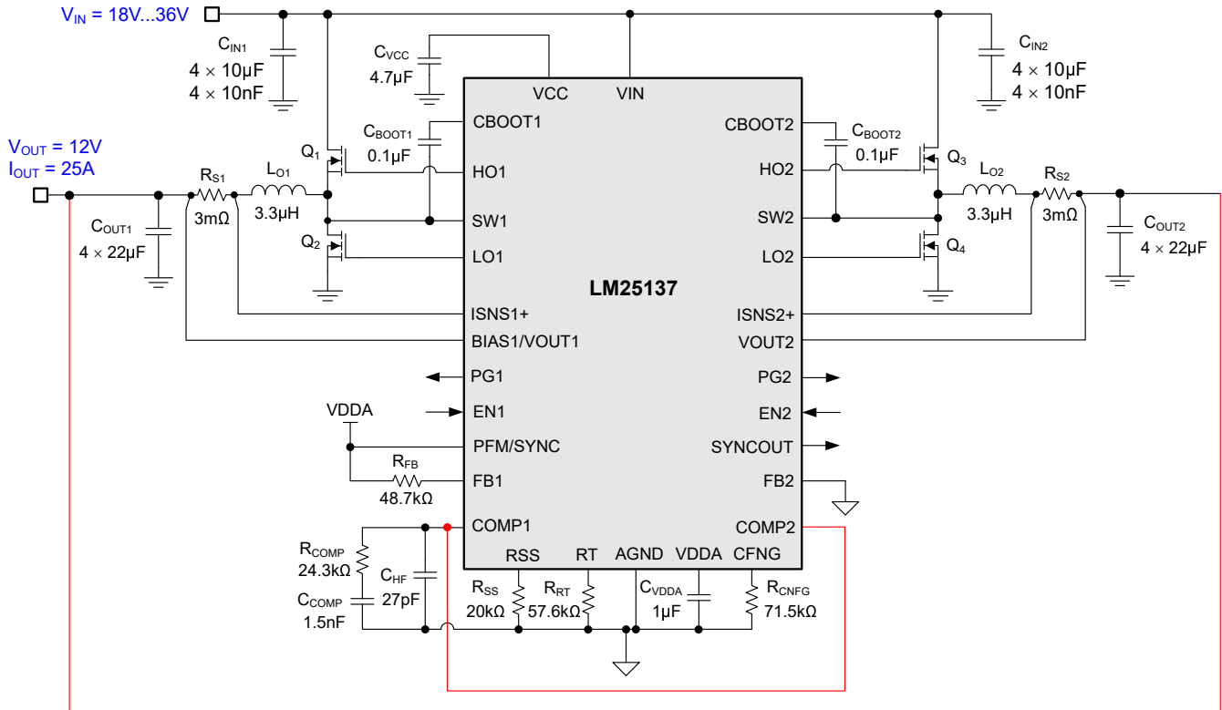
图 8-20. 采用 LM25137 两相降压稳压器且开关频率为 400kHz 时的应用电路 3
