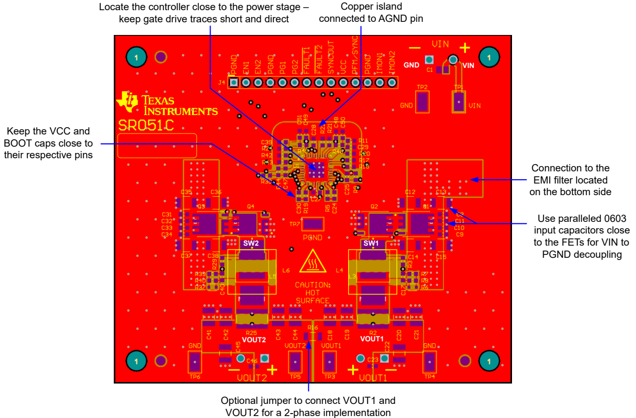
图 8-26. PCB 顶层
