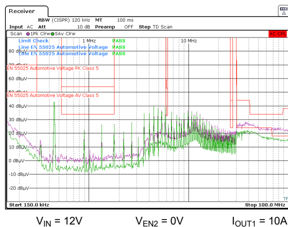
图 8-16. CISPR 25 5 类 EMI 性能，5V 10A 输出，禁用通道 2
