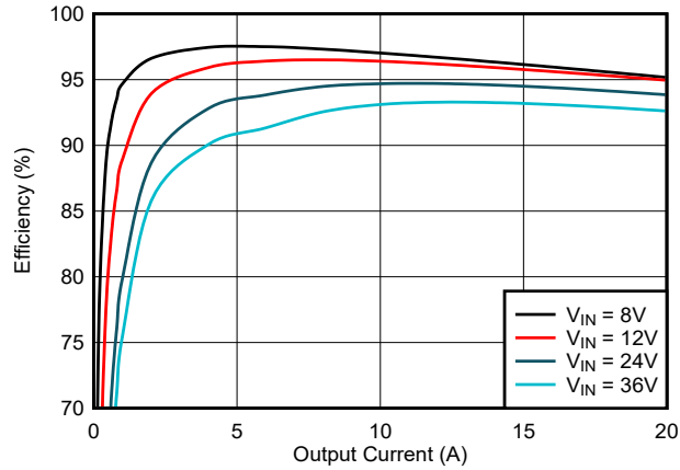
图 8-5. 效率与 I_{OUT1} 之间的关系
