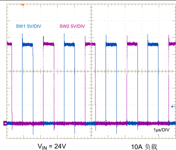
图 8-21. 开关节点电压
