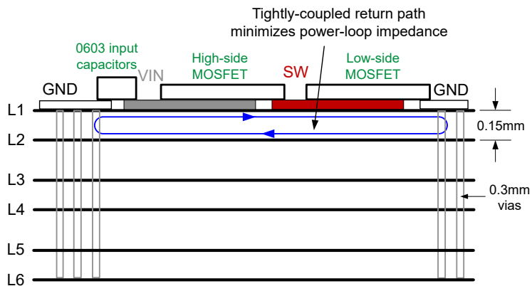
图 8-27. 功率级元件布局
