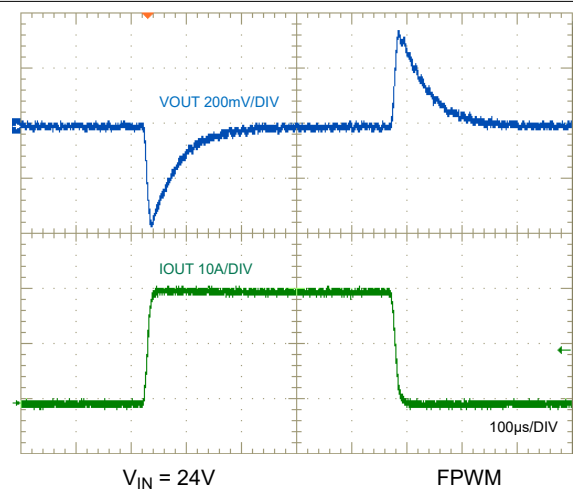
图 8-23. 负载瞬态, 0A 至 20A
