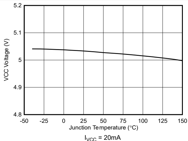
图 6-16. VCC 稳压电压与温度间的关系
