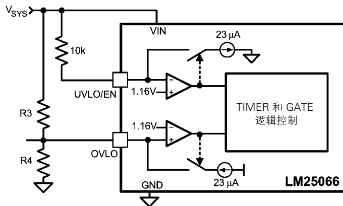
图 12: UVLO = POR
