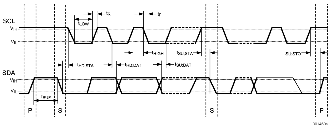
图 19: SMBus 时序图
