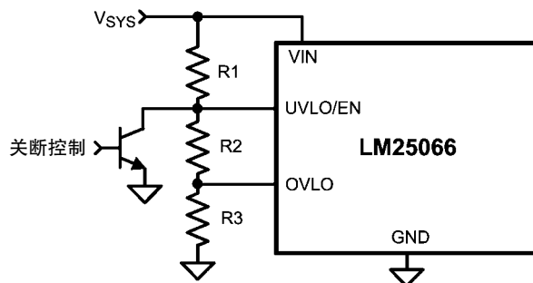
图 5：关断控制
