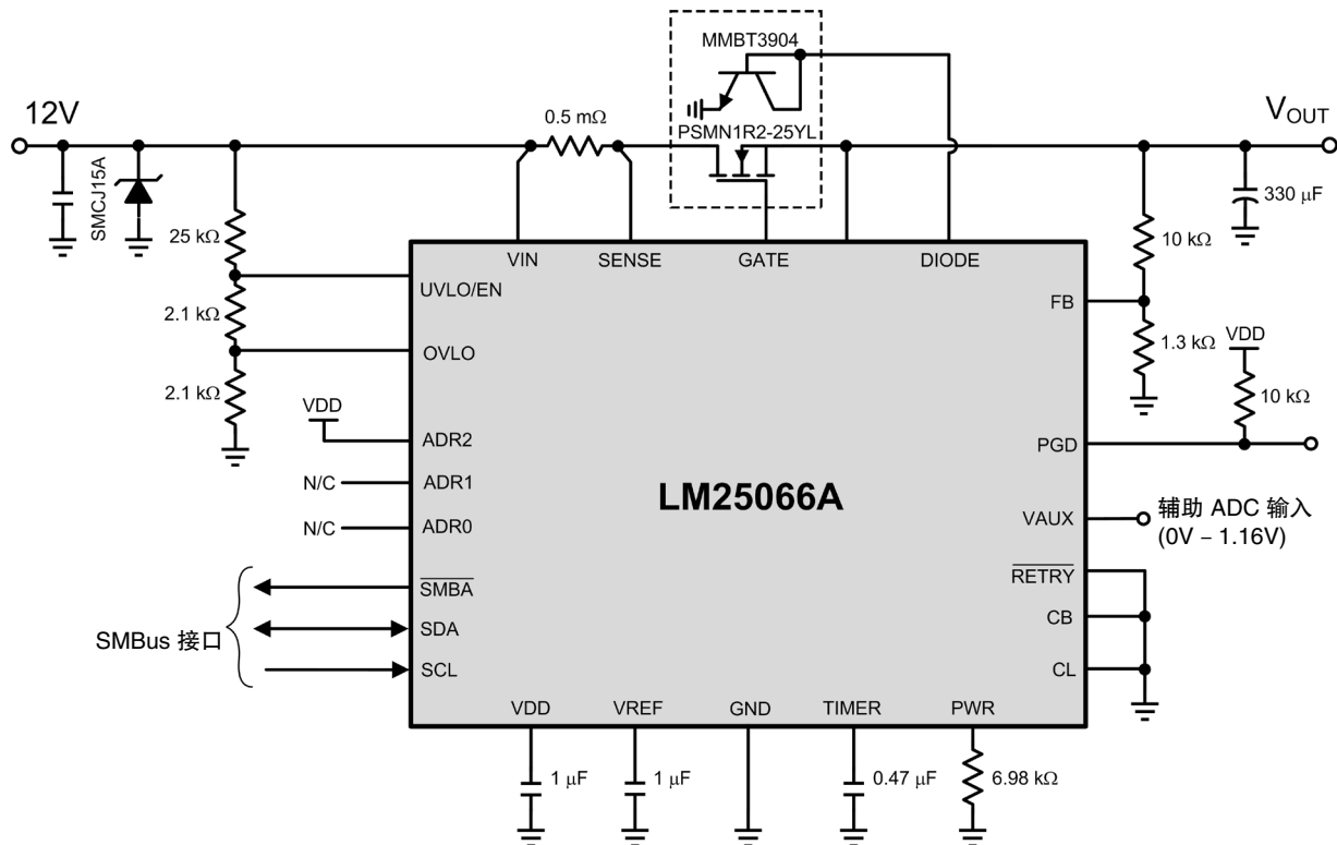
图 6：典型应用电路
