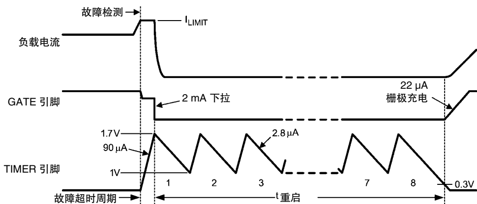
图 4：重启过程
