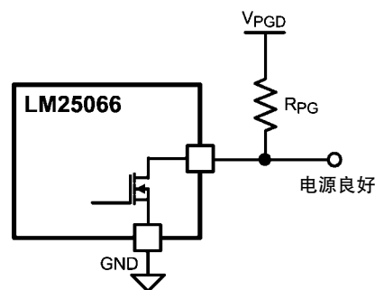
图 14: 电源良好输出
