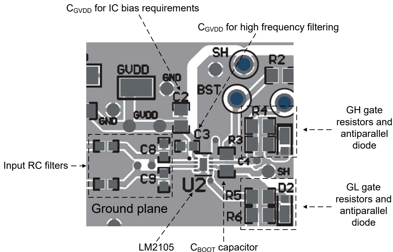
图 10-1. Layout Example
