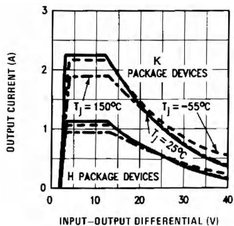
图 7-2. Current Limit
