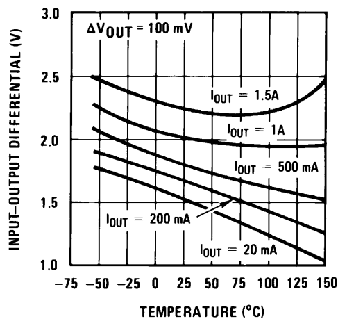
图 7-4. Dropout Voltage
