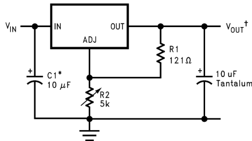
典型应用
