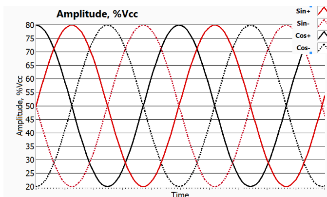
图 8-1. LDC5072-Q1 Typical Output
