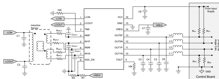
LDC5072-Q1 典型应用图
