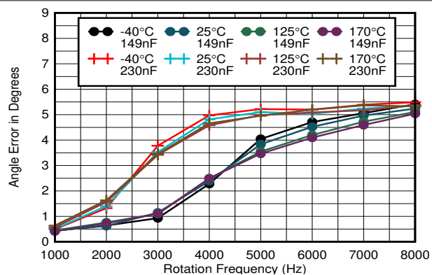
图 7-5. Angle Error VCC = 5 V, C OUT > 100 nF
