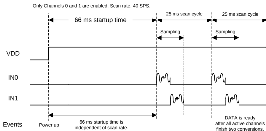
图 21. Power-On Timing
