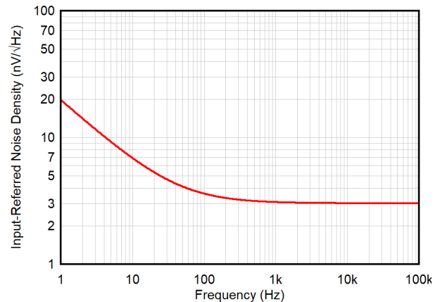
图 9-9. Input-Referred Noise Density
