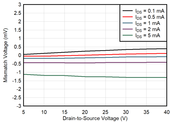
图 6-13. V_{GS} Mismatch vs V_{DS}
