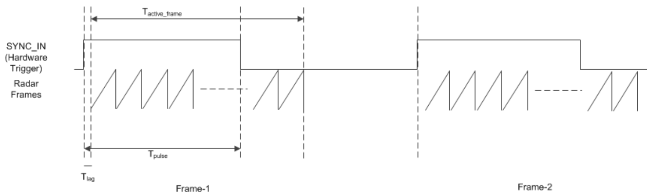
图 7-7. SYNC IN 硬件触发器
