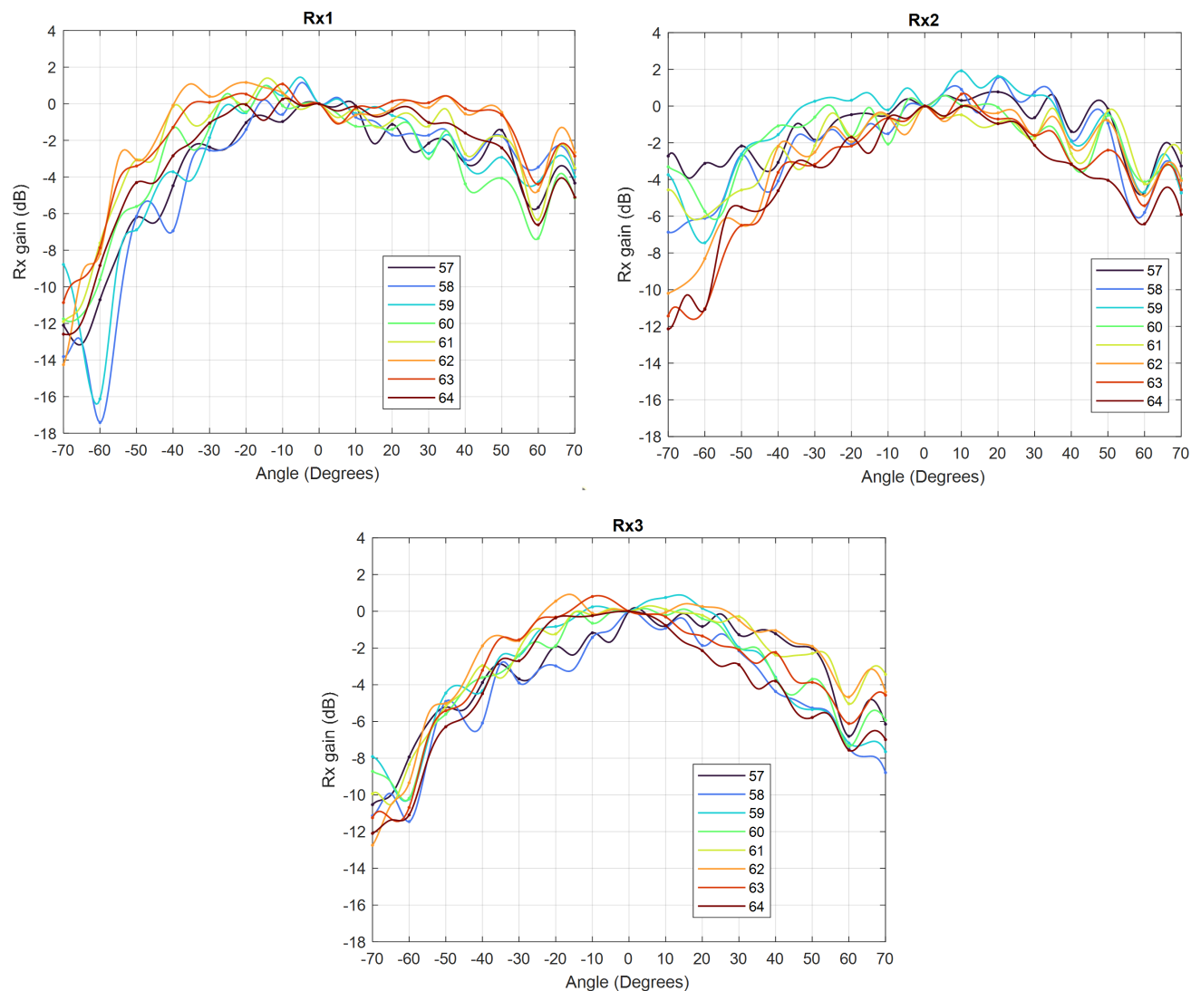
图 7-8. 接收器增益图标准化为视轴
