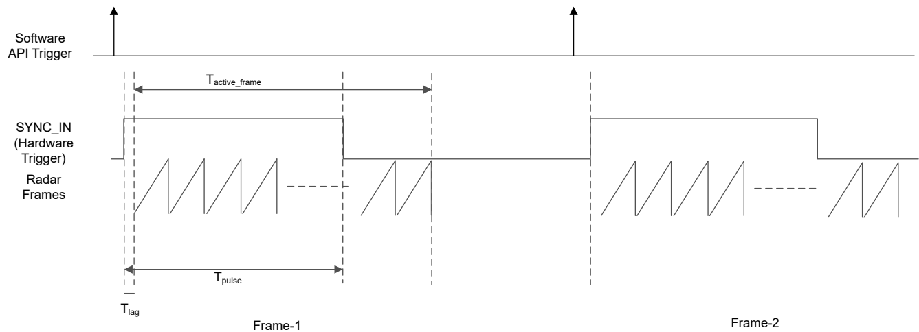
图 7-12. SYNC IN 硬件触发器
