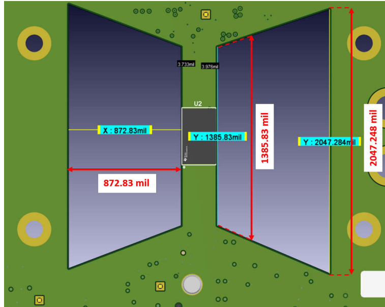
图 7-7. 具有梯形切口的大型电路板，PCB 边缘小于 0.3mm
