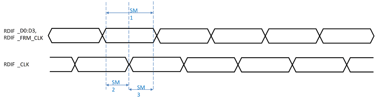
图 7-18. RDIF 时序要求
