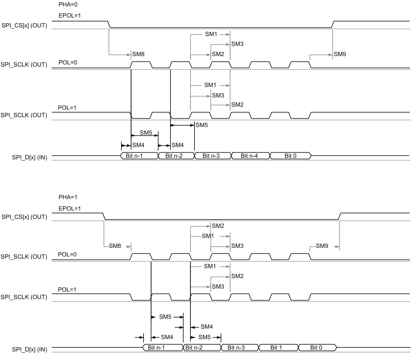
图 7-14. SPI 时序 — 控制器模式接收
