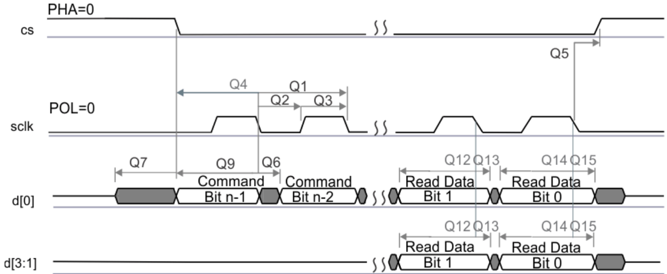
图 7-21. QSPI 读取 (时钟模式 0)
