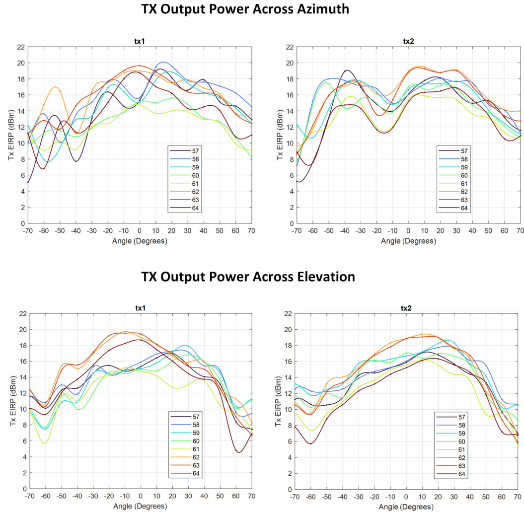
图 7-9. 发送器天线辐射方向图
