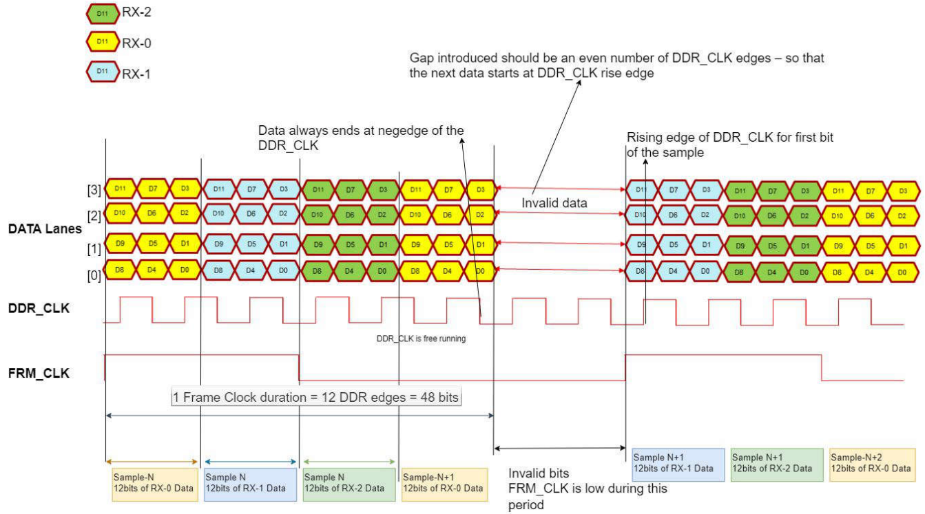
图 7-19. RDIF 数据格式
