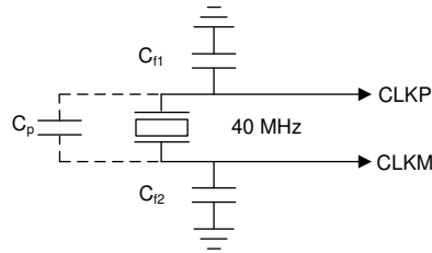
图 7-13. 晶体实现
