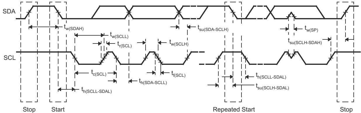
图 7-20. I2C 时序图
