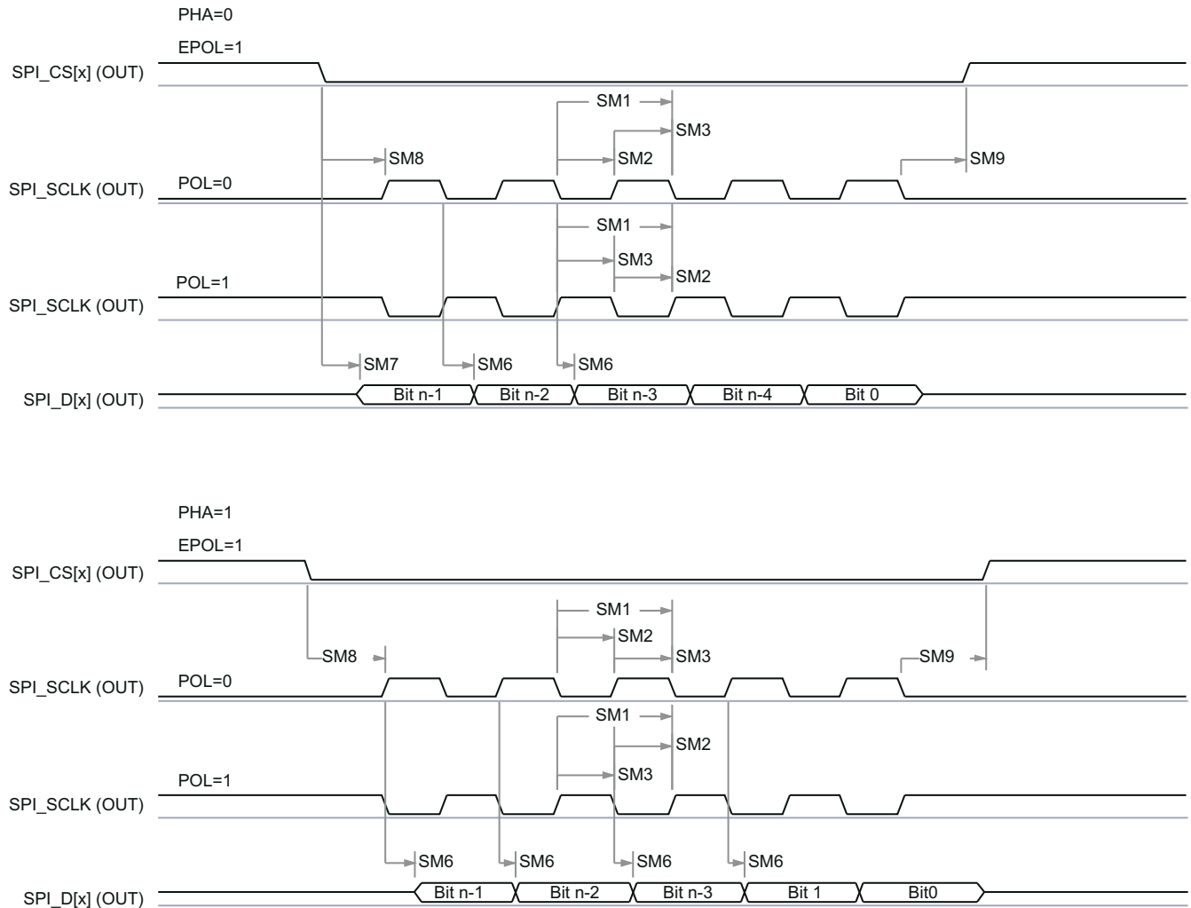
图 7-15. SPI 时序 — 控制器模式发送
