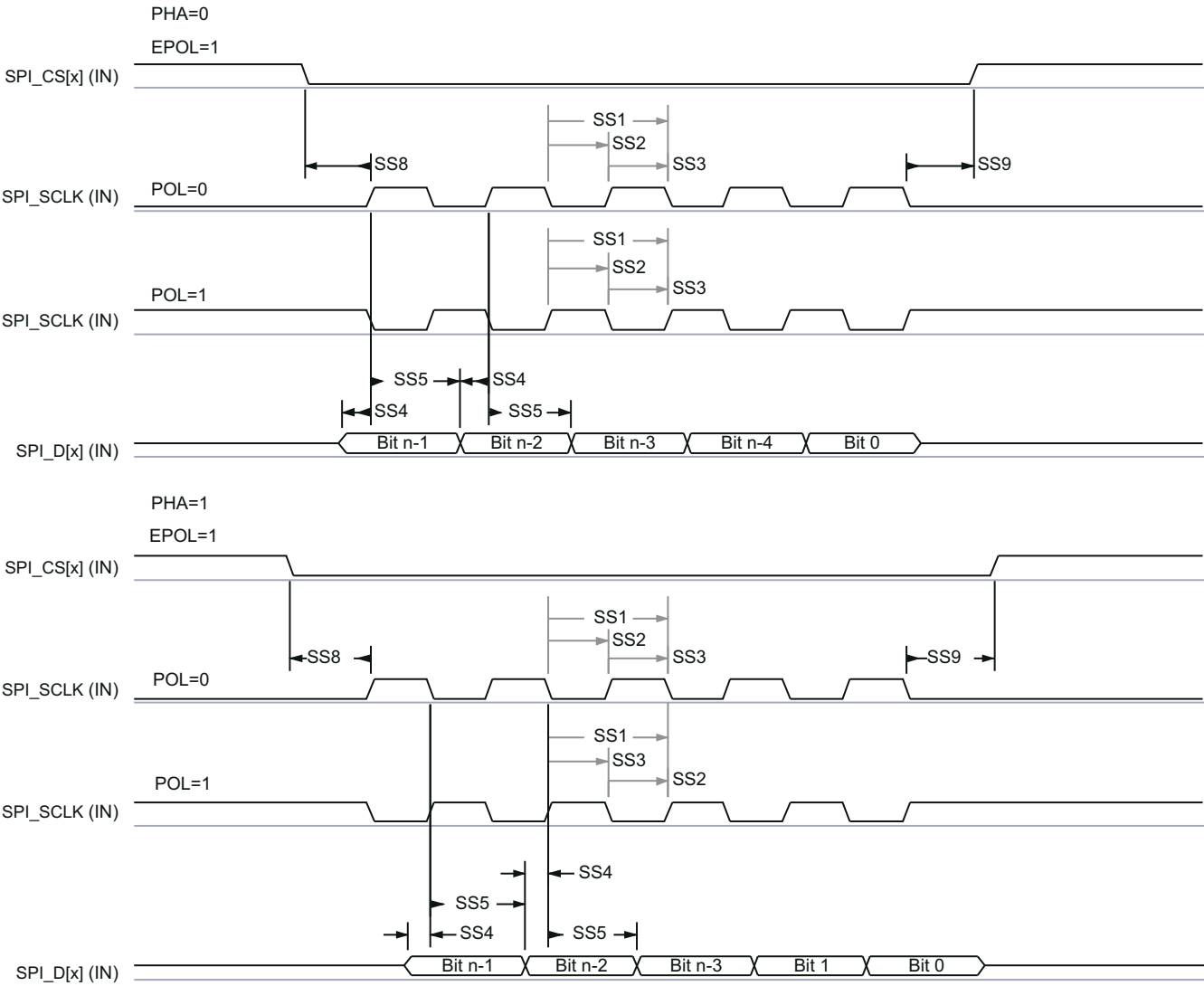
图 7-16. SPI 时序 — 外设模式接收
