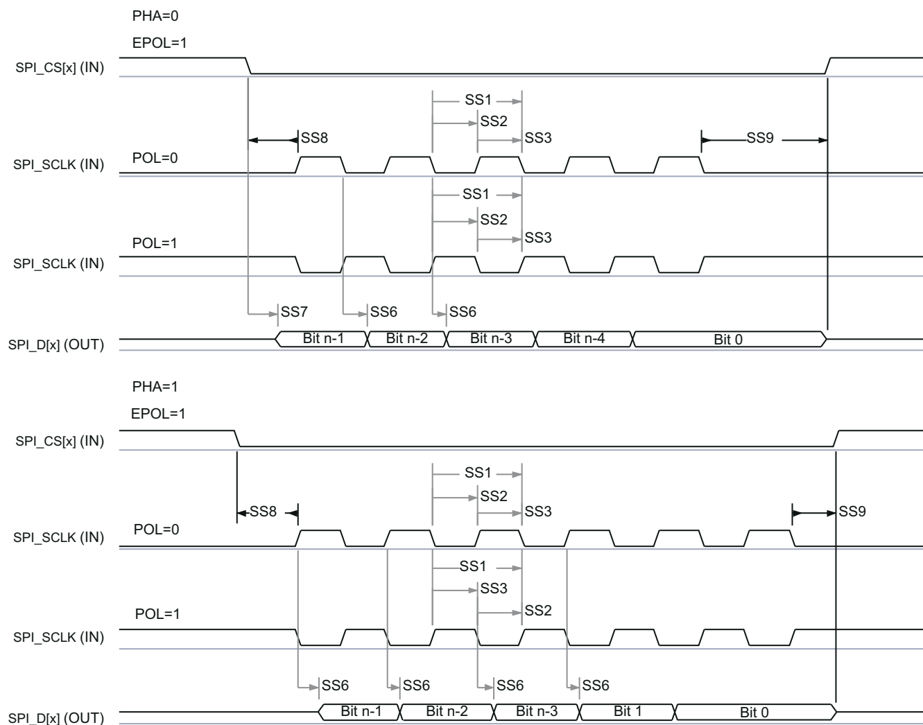
图 7-17. SPI 时序 — 外设模式发送
