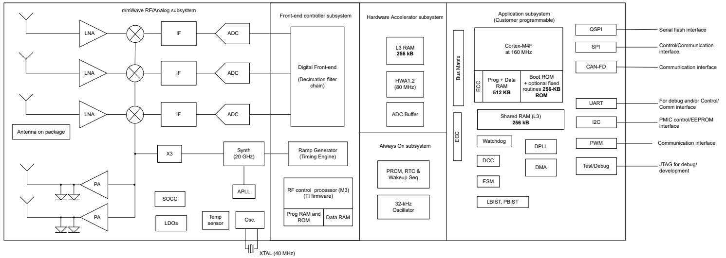
图 4-1. 功能方框图
