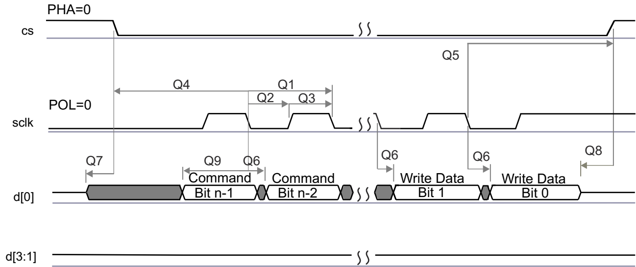
图 7-22. QSPI 写入 ( 时钟模式 0 )
