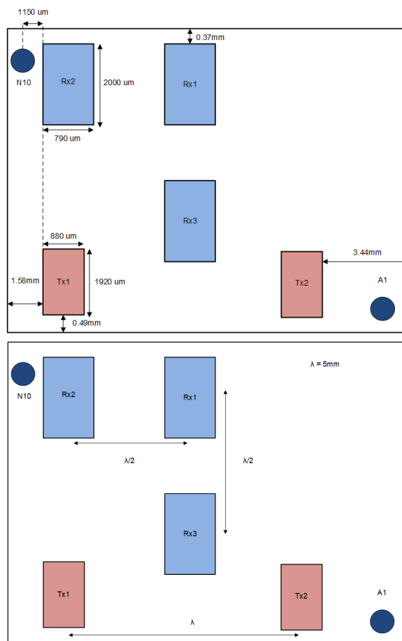
图 7-10. 天线位置 ( 放置和相对间距 )
