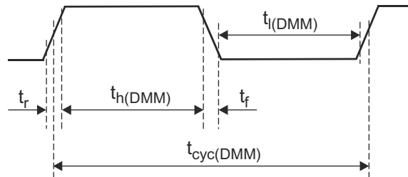
图 7-19. DMMCLK 时序
