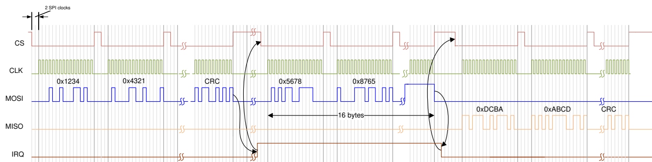
图 7-11. SPI 通信
