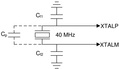
图 7-4. 晶体实现
