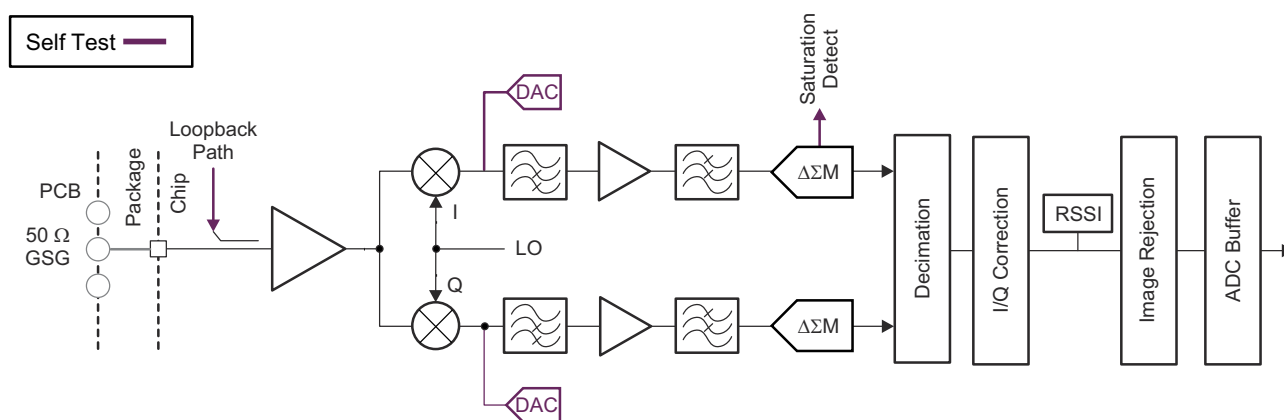
图 8-4. 接收子系统 (每通道)
