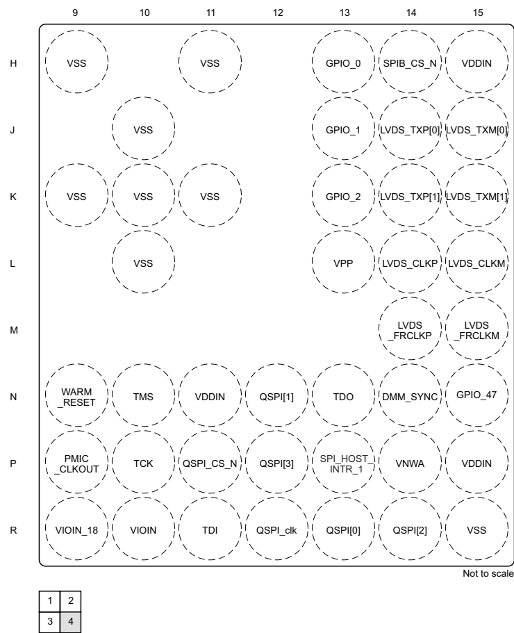
图 6-5. 右下象限
