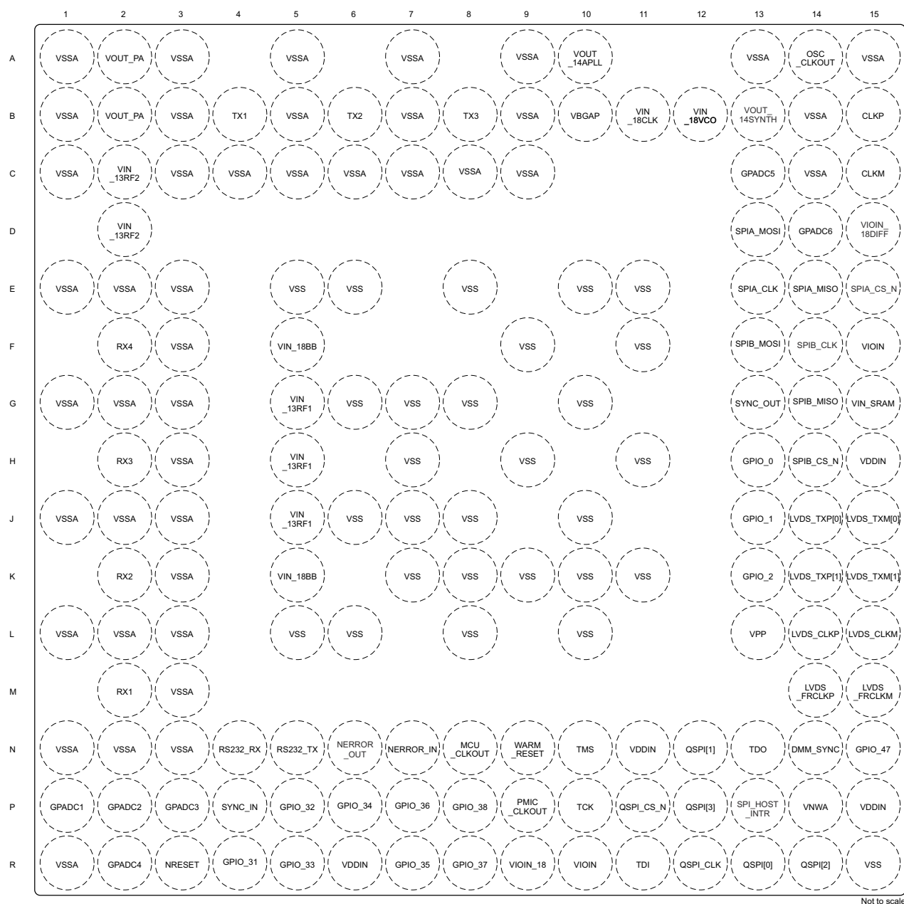
图 6-1. 引脚图
