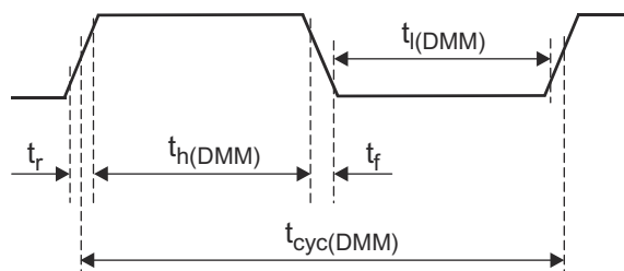
图 8-18. DMMCLK Timing
