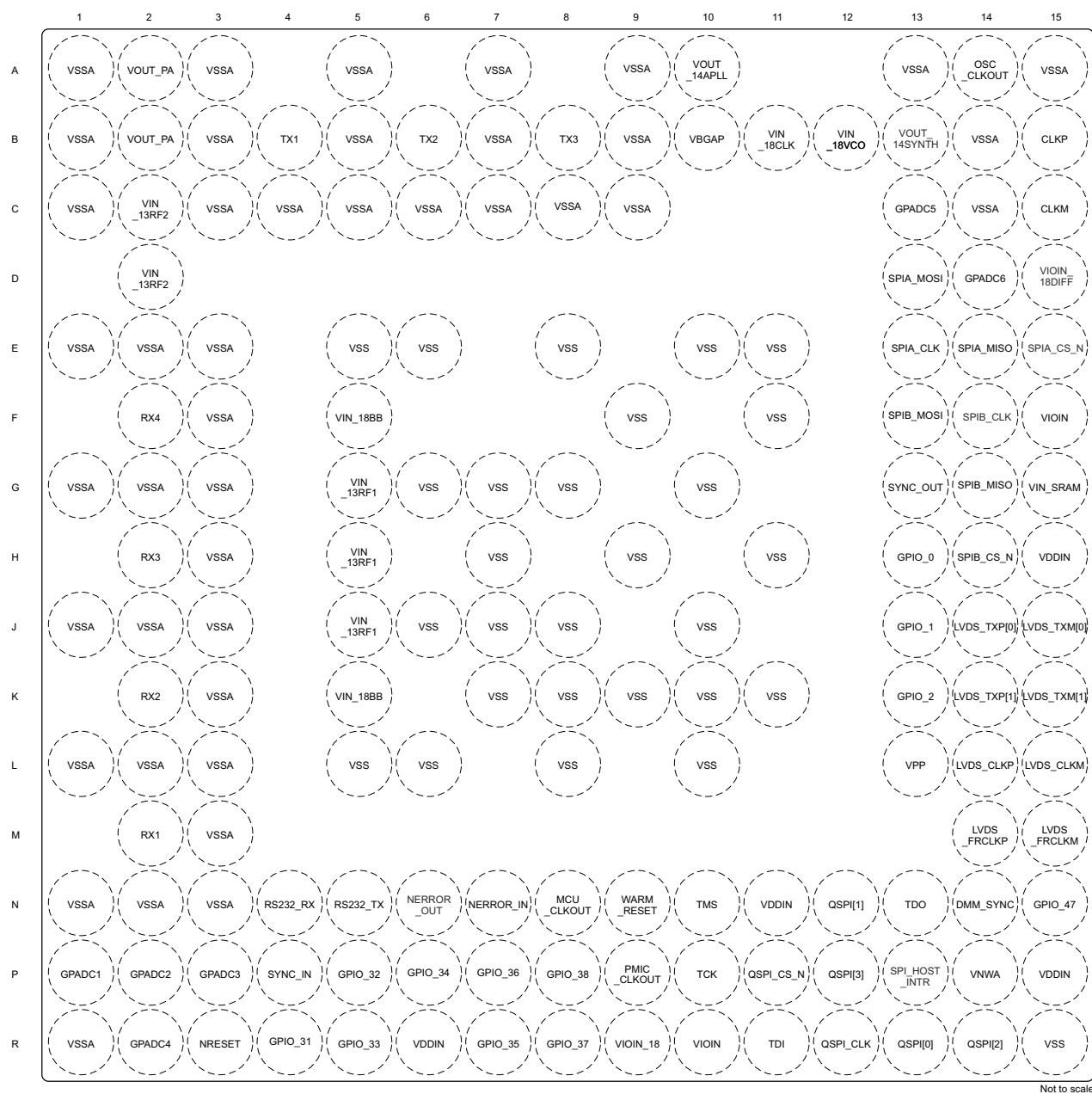
图 7-1. Pin Diagram
