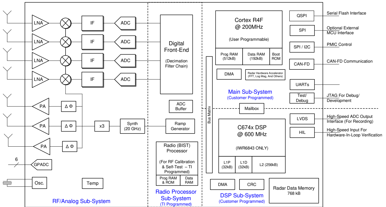
图 4-1. 功能方框图
