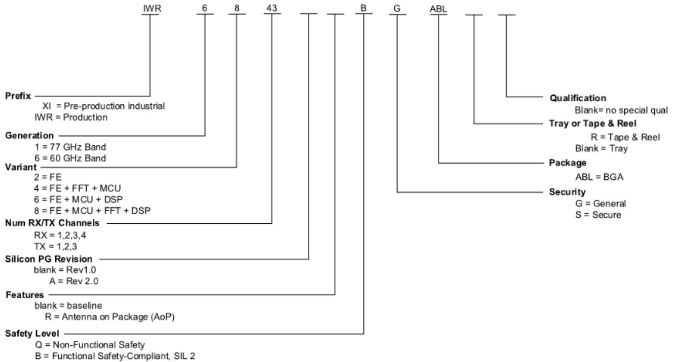
图 12-1. Device Nomenclature
