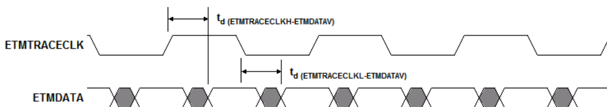
图 8-17. ETMDATA Timing
