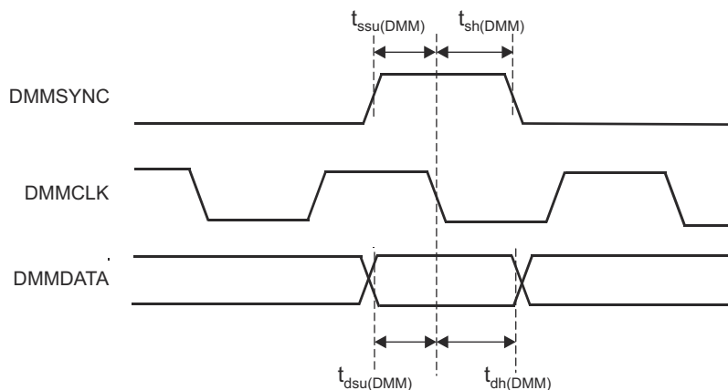
图 8-19. DMMDATA Timing
