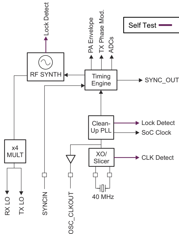
图 8-1. Clock Subsystem
