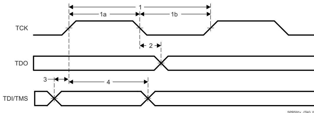
图 7-24. JTAG Timing
