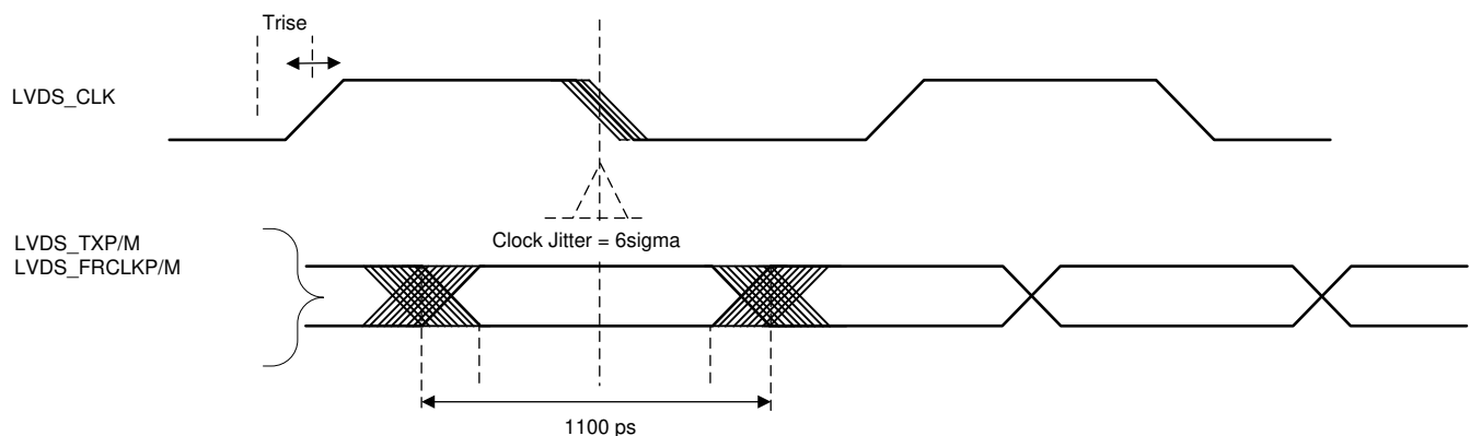
图 7-16. Timing Parameters
