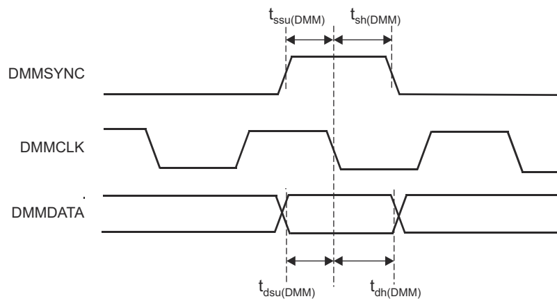
图 7-23. DMMDATA Timing
