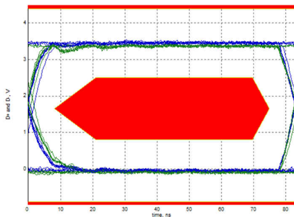
图 6-5. 通过 ISOUSB111 实现的典型全速 (12Mbps) 眼图
