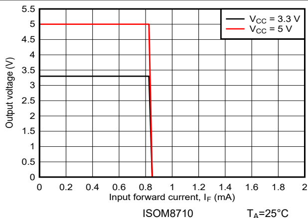
图 7-3. 输出电压与输入正向电流间的关系
