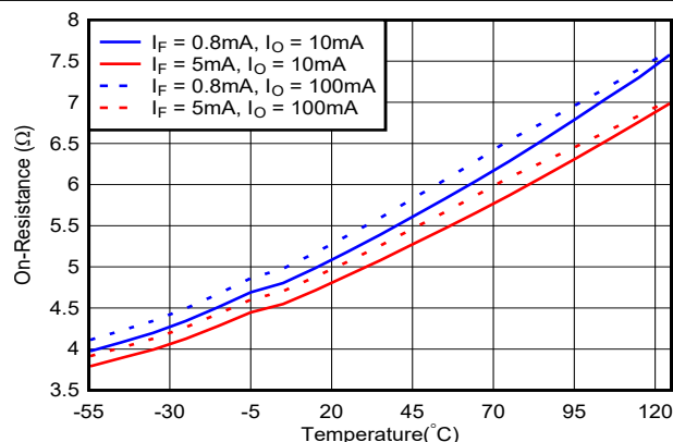
图 6-5. 导通状态电阻与环境温度间的关系
