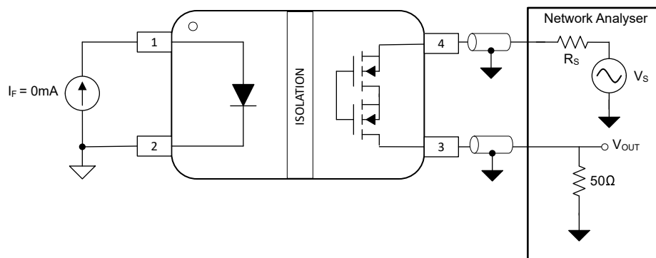
图 7-5. ISOM8610 关断状态隔离测试电路
