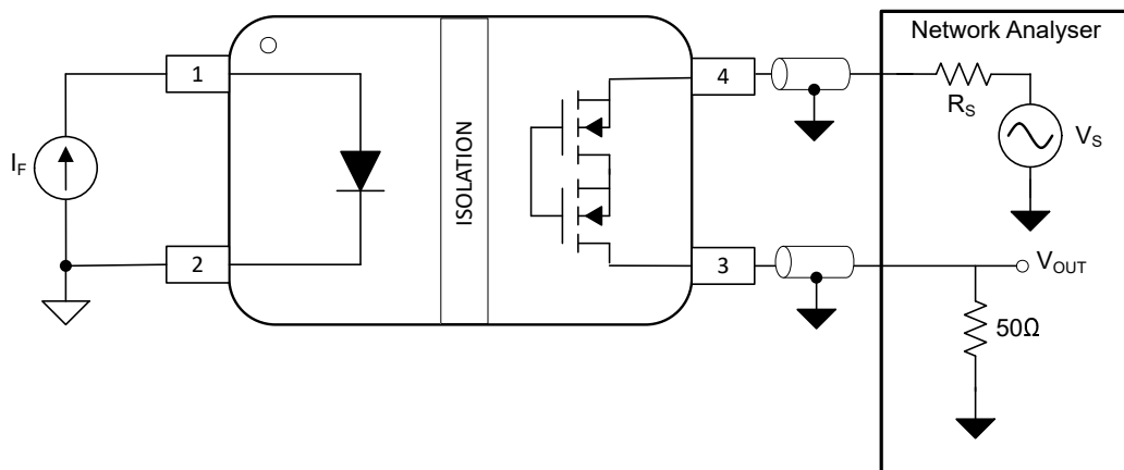
图 7-4. ISOM8610 插入损耗测试电路
