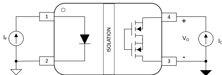
图 7-3. ISOM8610 导通状态电阻测试电路
