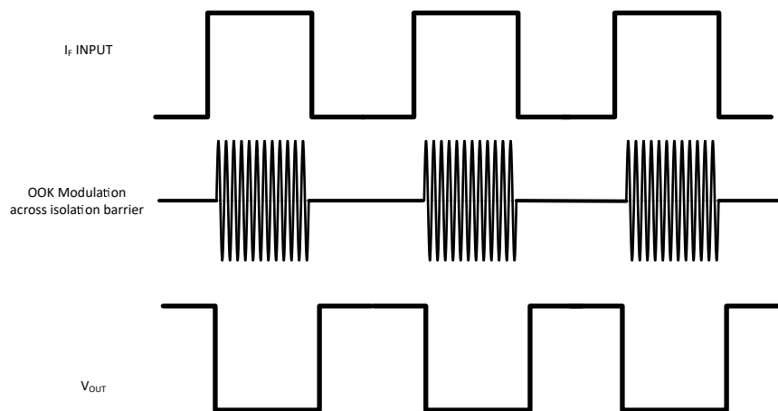
图 8-2. 基于开关控 (OOK) 的调制方案
