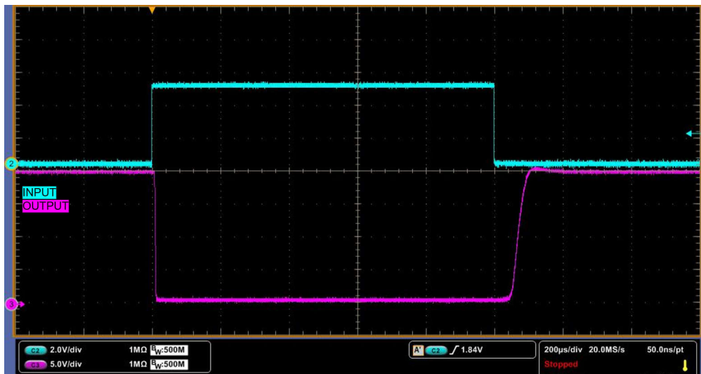
图 9-2. I_F = 5mA 、 V_{CC} = 20V 、 R_L = 200\Omega 且 C_L = 50pF 时的典型波形
