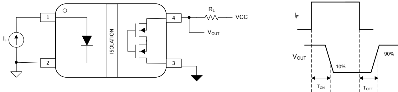
图 7-1. ISOM8610 导通和关断时间测试电路
