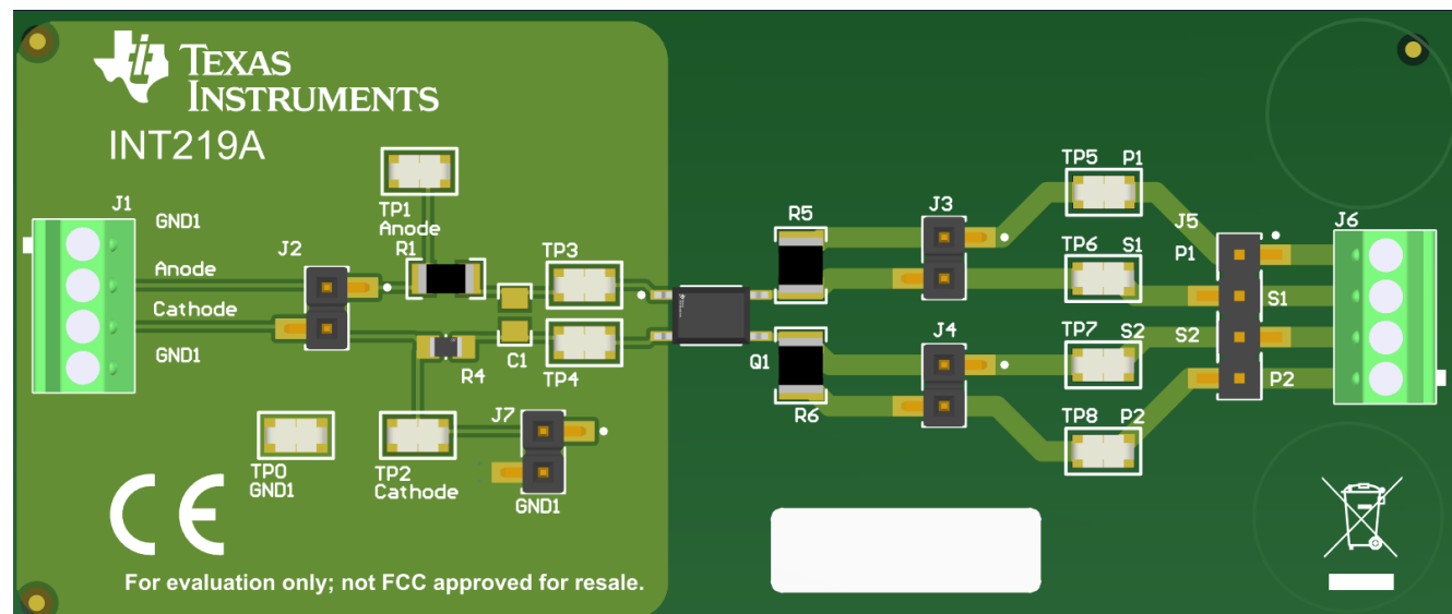
图 9-3. 采用 2 层电路板的 ISOM8610 布局示例
