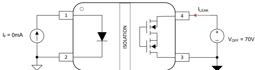
图 7-2. ISOM8610 关断状态漏电流测试电路
