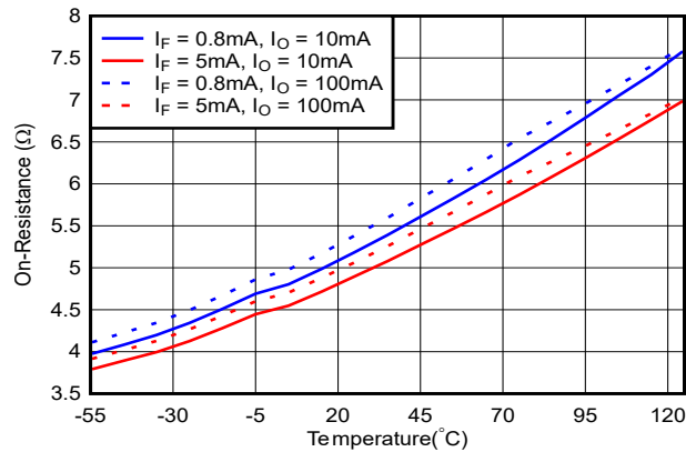
图 6-5. 导通状态电阻与环境温度间的关系
