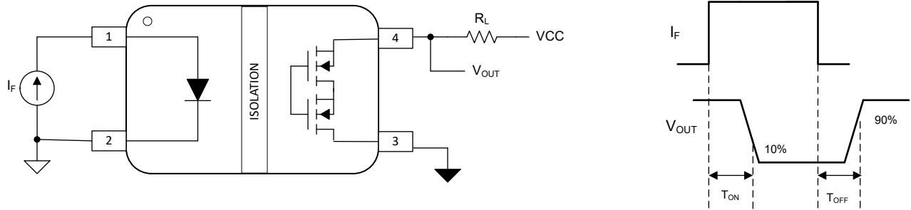
图 7-1. ISOM8600 导通和关断时间测试电路
