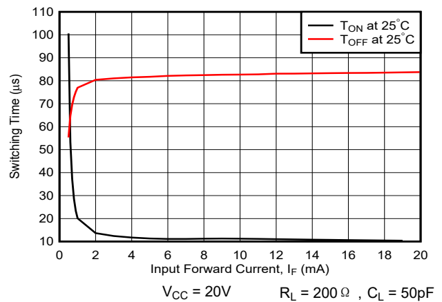
图 6-8. 导通和关断时间与正向电流间的关系
