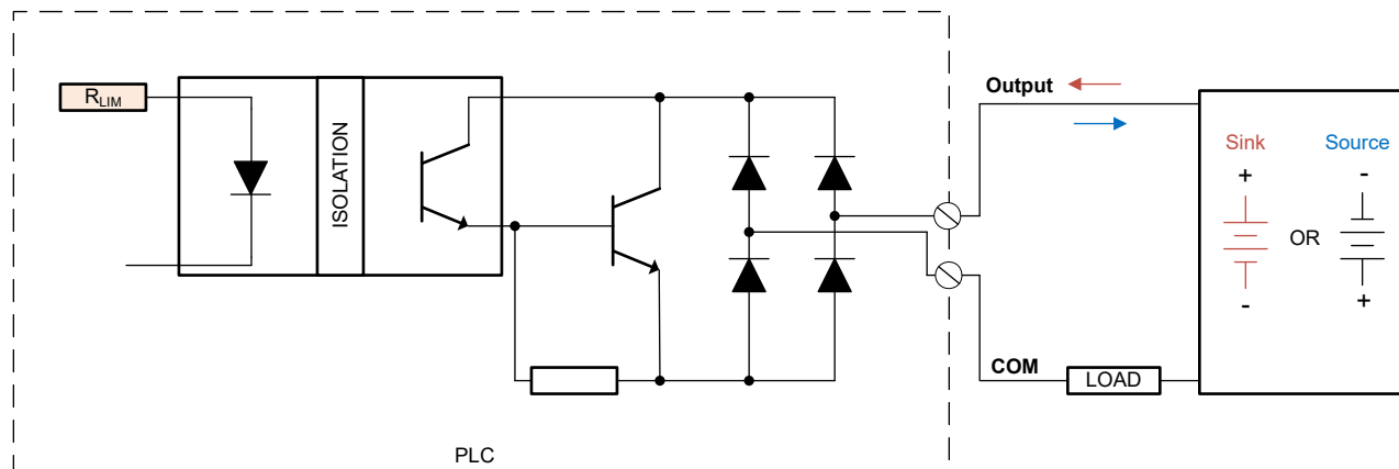
图 9-1. 采用分立式实施的典型数字输出级
