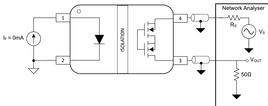
图 7-5. ISOM8600 关断状态隔离测试电路
