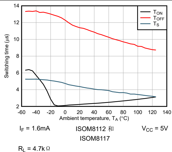
图 6-28. 开关时间与环境温度间的关系
