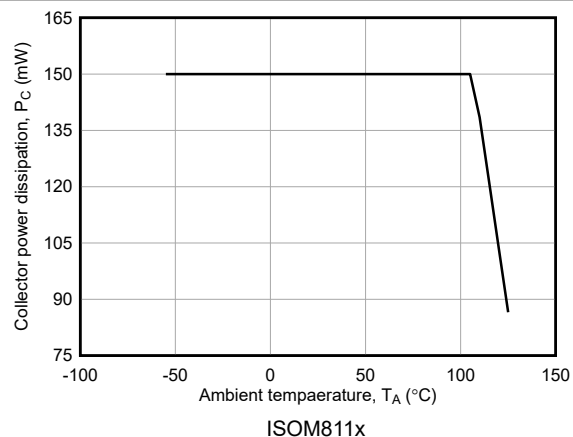
图 6-2. 最大集电极功率耗散与环境温度间的关系
