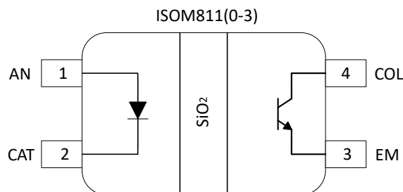
图 5-1. ISOM811[0-3] 4 引脚 SOIC (顶视图)
