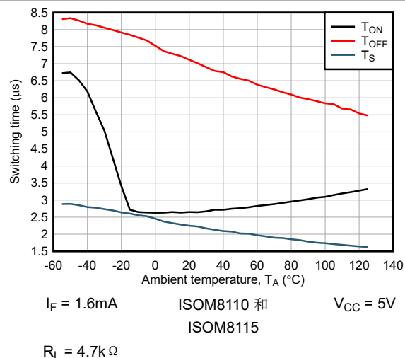
图 6-26. 开关时间与环境温度间的关系
