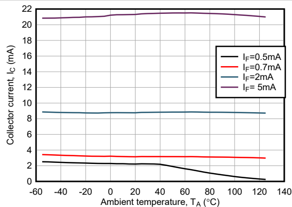
图 6-19. 集电极电流与环境温度间的关系
