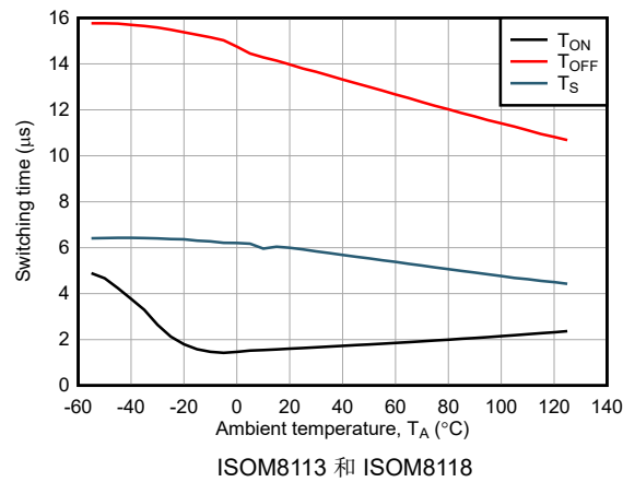
图 6-27. 开关时间与环境温度间的关系
