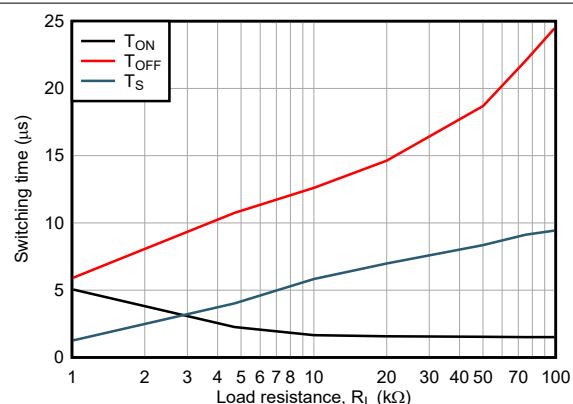
图 6-22. 开关时间与负载电阻间的关系
