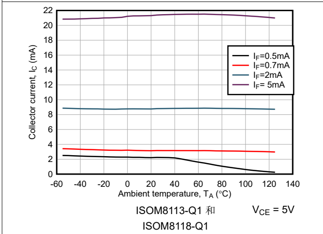
图 6-21. 集电极电流与环境温度间的关系
