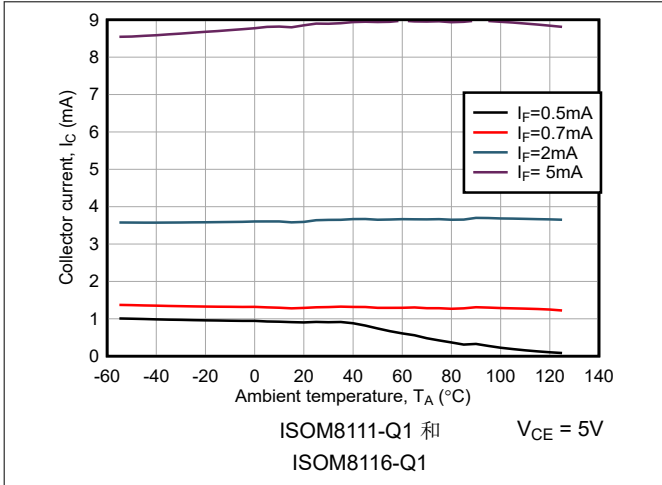
图 6-19. 集电极电流与环境温度间的关系
