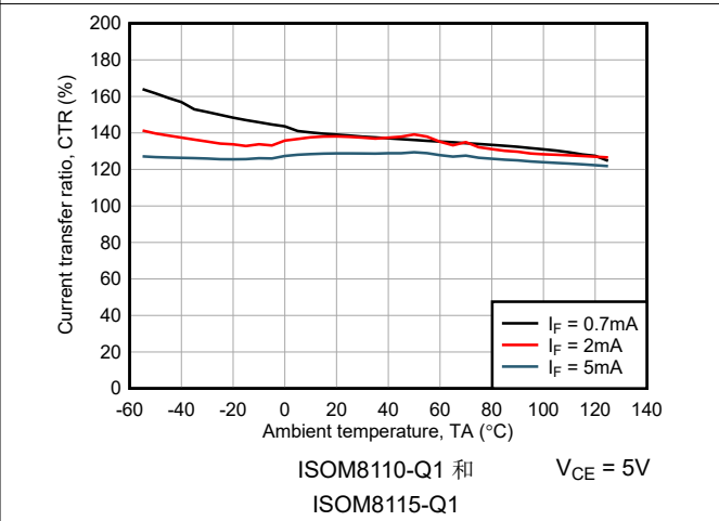
图 6-22. 电流传输比与环境温度间的关系
