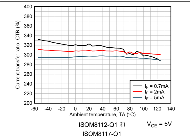
图 6-24. 电流传输比与环境温度间的关系
