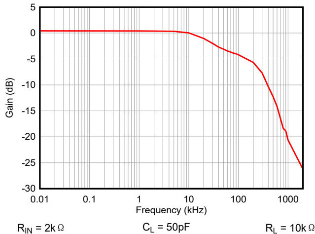
图 9-6. R_L = 10k\Omega 时的带宽
