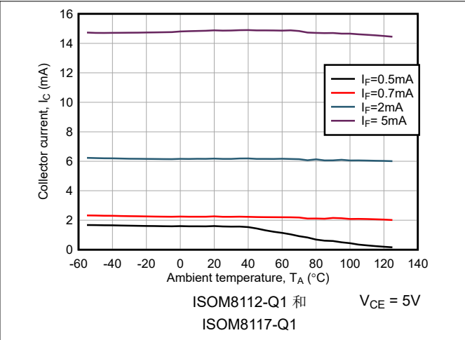
图 6-20. 集电极电流与环境温度间的关系
