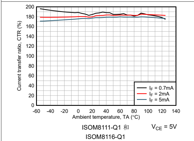
图 6-23. 电流传输比与环境温度间的关系
