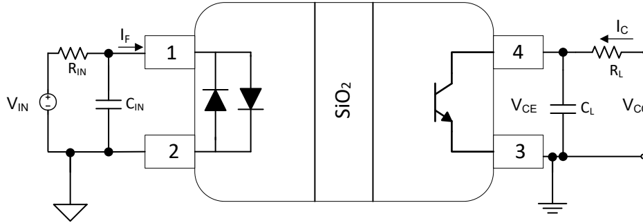
图 7-5. ISOM811[5-8]-Q1 带宽测试电路
