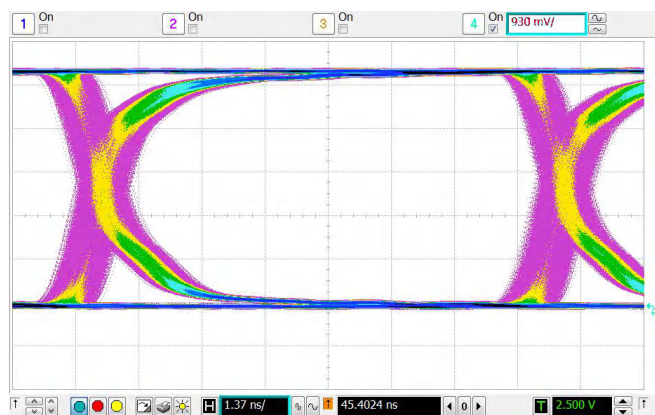
图 8-3. 眼图：100Mbps PRBS、5V 和 25°C
