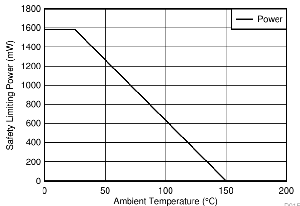
图 5-4. 根据 VDE 标准限制功率的热降额曲线
