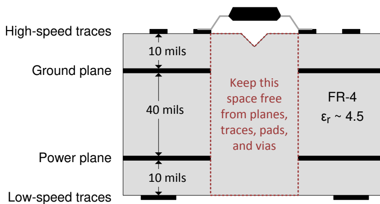
图 8-4. Layout Example
